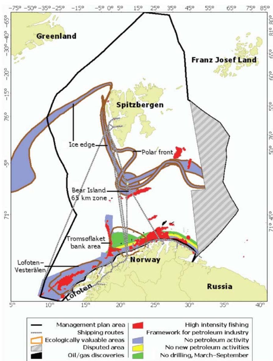
Figur 27. Areal, som er omfattet af forvaltningsplanen for Barentshavet, som viser primære fiskeområder, skibsruter samt afgrænsede områder til olieeftersforskning sammen med særligt værdifulde og følsomme områder. Figur fra Olsen et al. (2007).
