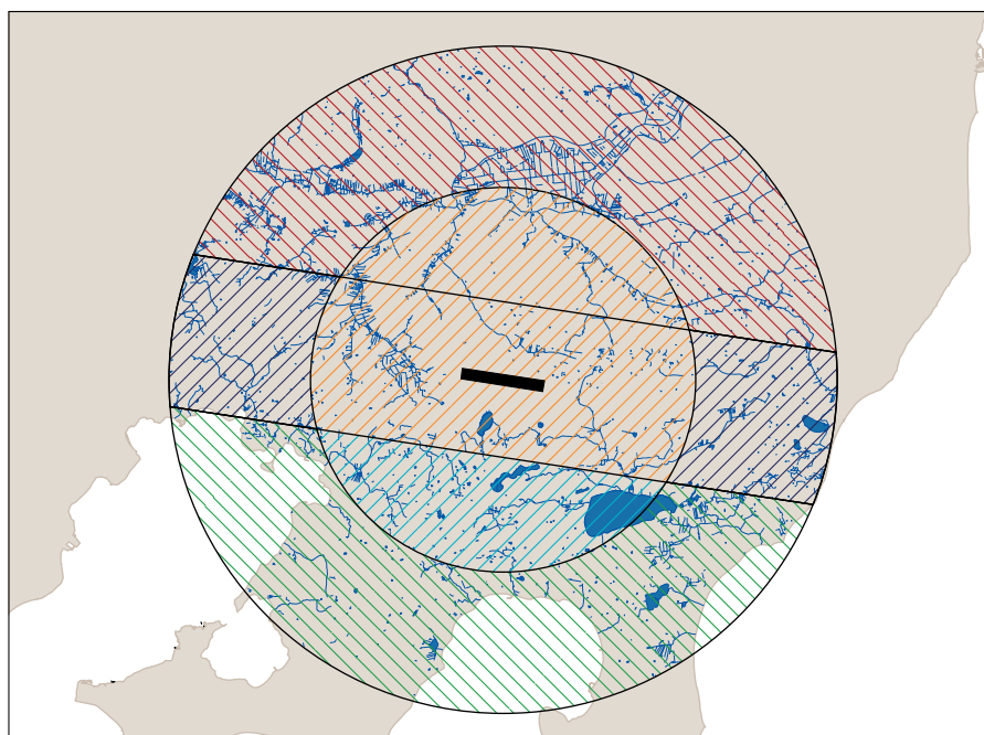
Figur 16. Placering af Århus Lufthavns landingsbane og 6 km (radius 7,5 km) og 13 km afstands zoner. En zone på 6 km's bredde parallelt med landingsbanerne er tilsvarende indtegnet. Søer og vandløb registreret i Miljø- og Energiministeriets Areal Informations System (AIS) pr. 31. 12. 2004 er vist inden for 13 km zonen.
