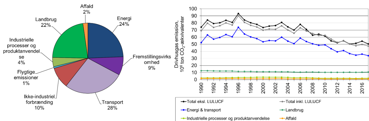
Figur S.1 Danske drivhusgasemissioner. Bidrag til total emission fra hovedsektorer for 2017 og tidsreier i CO 2 -ækvivalenter for 1990-2017, hvor data er angivet med og uden LULUCF.
