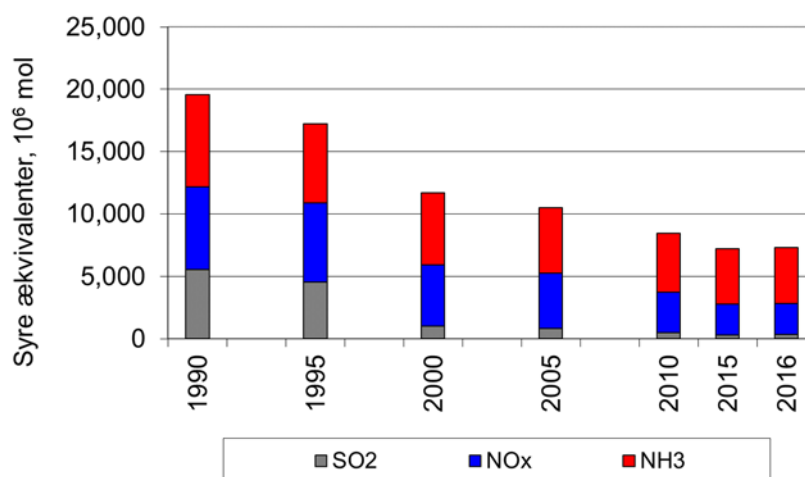
Figur 1.1 Emissioner af NH 3 , NO x og SO 2 i syreækvivalenter.
