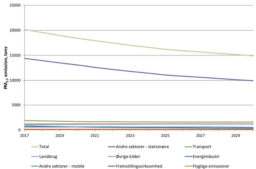
Figur 3.5 Udviklingen i \text{PM}_{2,5} -emission i WAM-fremskrivningen.
