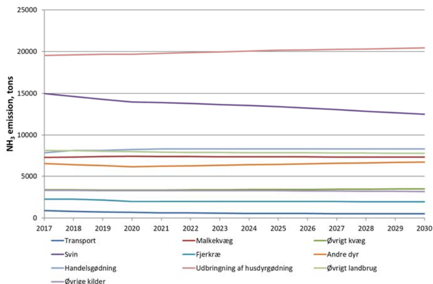
Figur 2.4 Basisfremskrivning af NH 3 .
