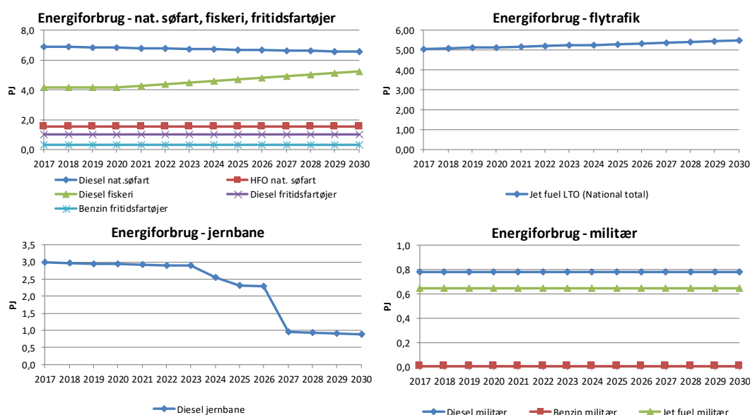
Figur 2.16 Energiforbruget for national søfart, fiskeri og fritidsfartøjer, flytrafik, jernbane og militær fra 2017-2030.
