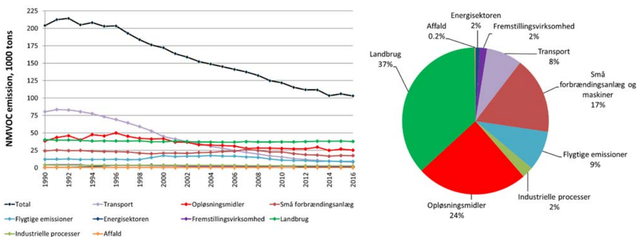
Figur 1.5 NMVOC-emissioner. Fordeling på hovedsektorer (2016) og tidsserien for 1990 til 2016.
