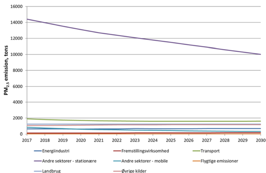
Figur 2.5 Basisfremskrivning af PM 2,5 .
