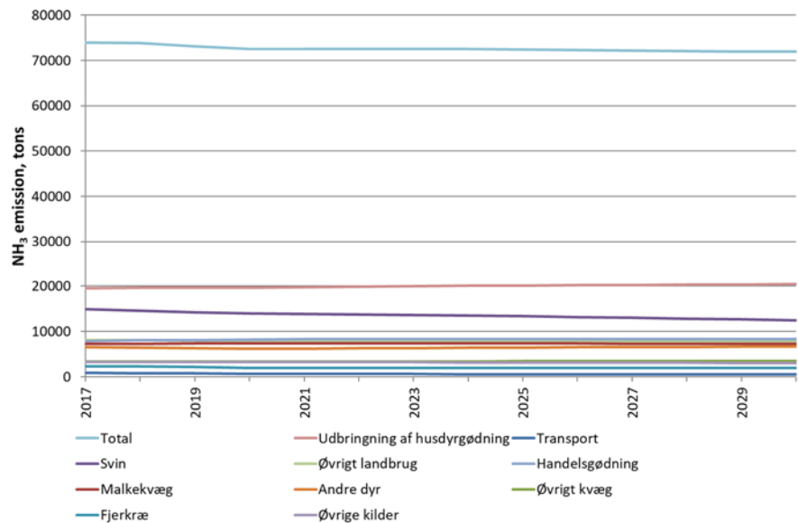
Figur 3.4 Udviklingen i \text{NH}_3 -emission i WAM-fremskrivningen.
