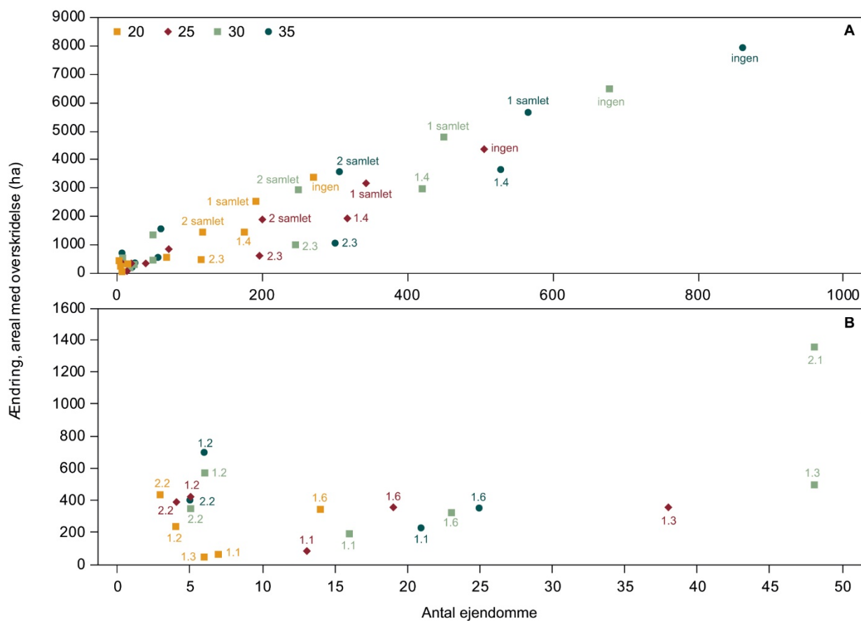
Figur 9. Ændring i areal med overskridelse af tålegrænserne (ha) som funktion af antal berørte ejendomme for de forskellige modeller for ændring af den specifikke ammoniakregulering
