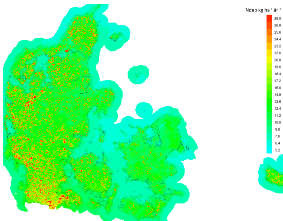
Figur 4. total kvælstofdeposition beregnet pba. baggrundsdeposition for 2005 – 2015 beregnet på 5,6 x 5,6 km 2 net og bidraget fra fuldtidslandbrug, 2015 som illustreret på figur 2.
