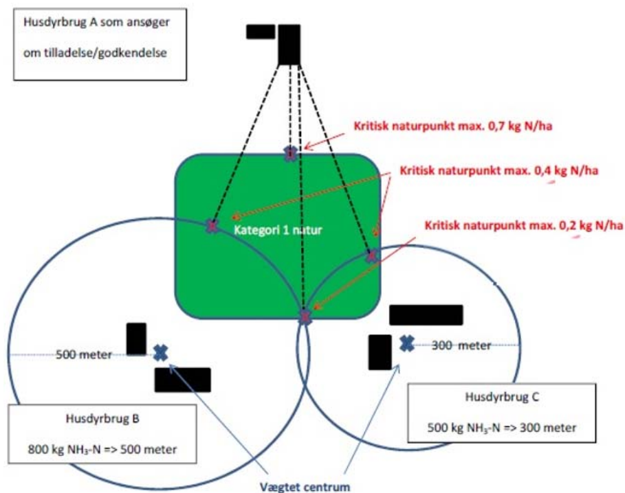
Figur 5. Kumulationsprincippet og kritiske naturpunkter for kategori 1 natur 9
