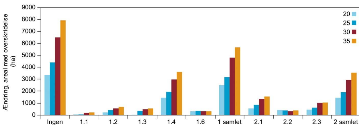
Figur 8. Ændring ift. baseline (nugældende specifikke ammoniakregulering) af hhv. areal med overskridelse af tålegrænsen (ha) for de forskellige modeller for ændring af den specifikke ammoniakregulering fordelt på årene 2020, 2025, 2030 og 2035, herunder også et scenarie med 'ingen' specifik ammoniakregulering.
