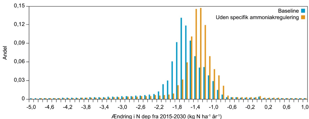
Figur 11. Beregnet fordeling i ændring af kvælstofbelastning fra 2015 til 2030 for baseline scenariet (blå) og et scenario uden specifik ammoniakregulering. Fordelingerne summerer til 1 og værdierne på y-aksen kan konverteres til % ved at gange med 100.
