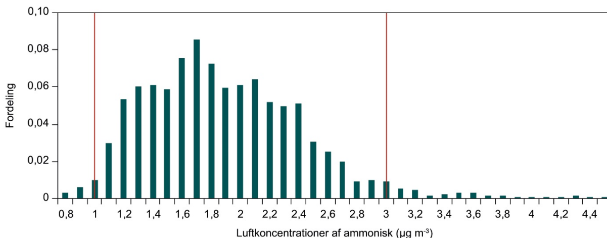
Figur 10. Fordelingen af danske luftkoncentrationer af ammoniak for kat 1, 2 og 3 fraregnet skov. ( \mu\text{g m}^{-3} , årlig gennemsnit beregnet for perioden 2005 – 2015, appendiks 3). UNECE anbefalede grænseværdier for mosser og laver ( 1 \mu\text{g m}^{-3} ) og højere planter ( 3 \mu\text{g m}^{-3} ) er indtegnet med rødt. Fordelingen summerer til 1 og værdierne på y-aksen kan konverteres til % ved at gange med 100.
