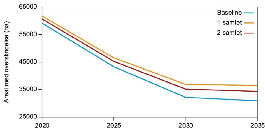
Figur 12. Tidsmæssigt forløb i udviklingen i areal med overskridelse af tålegrænsen for den ikke kantpåvirkede del af kategori 1, 2 og 3 natur fraregnet kategori 3 skov, for hhv. baseline scenariet og model 1 og 2, samlet.
