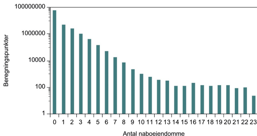
Figur 7. Antal naboejendomme, der bidrager til afsætning med gældende definition fordelt på naturarealet. Et beregningspunkt er 50 x 50 m 2 .
