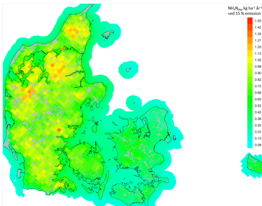
Figur 3. Forøgelse af deposition af dansk ammoniak ved 15 % forøget \text{NH}_3 -emission. Depositionsforøgelsen er størst i Jylland, specielt i Nordvestjylland.
