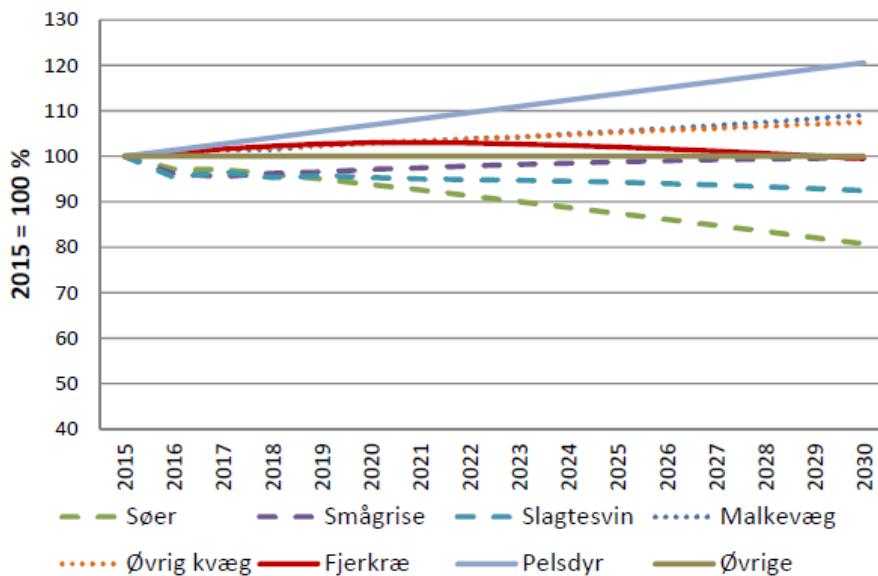
Figur A2.1. Udvikling i antallet af husdyr i fremskrivning af ammoniak.
