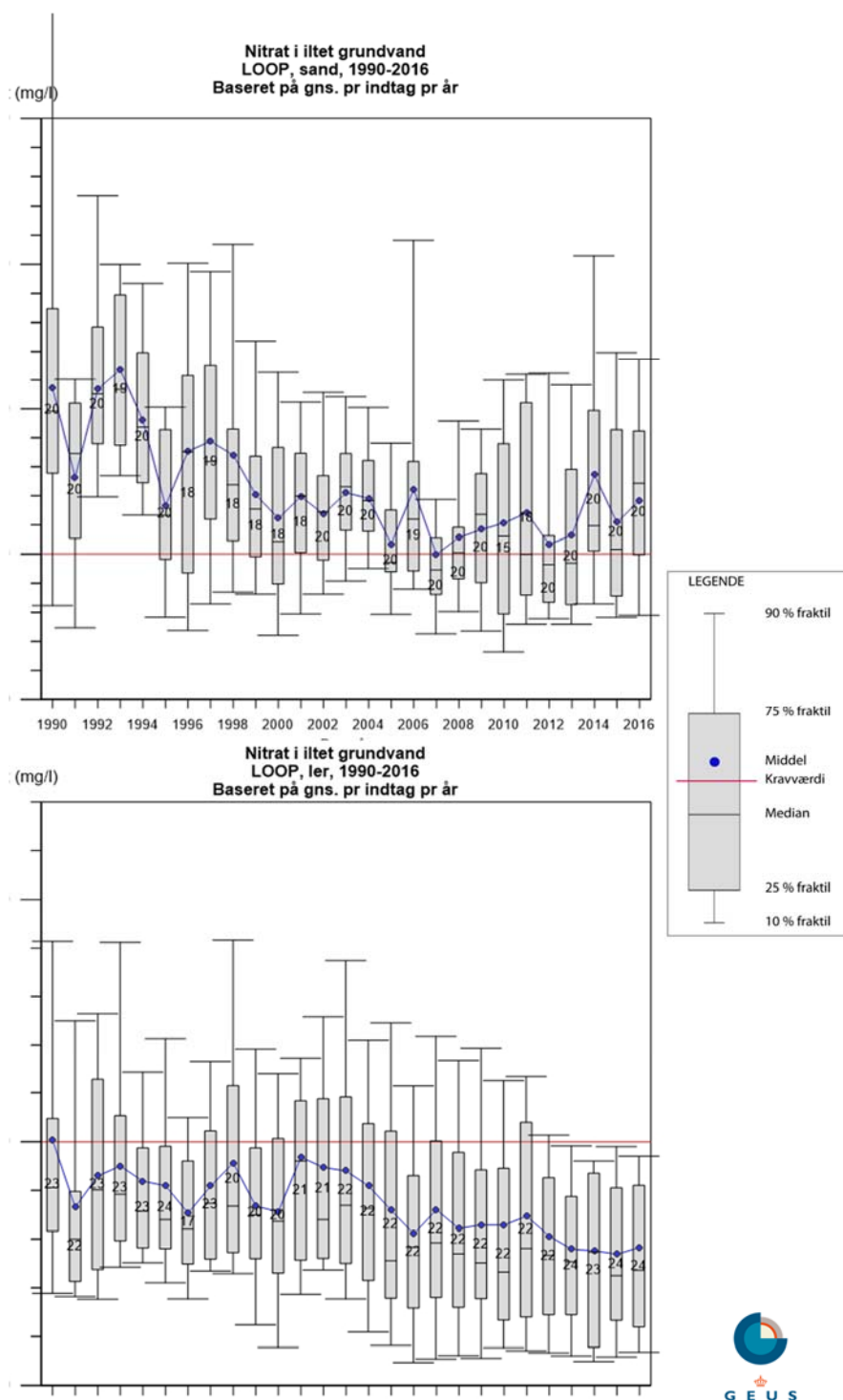
Figur 4.10. Udviklingen i det ilt-holdige grundvands nitratindhold i LOOP-område med sand (LOOP 2 og 6) og ler (LOOP 1, 3 og 4) vist som boksdiagrammer for hvert kalenderår i perioden 1990-2016. Diagrammet er baseret på det gennemsnitlige nitratindhold pr. indtag. Antallet af indtag er angivet for hvert år.
