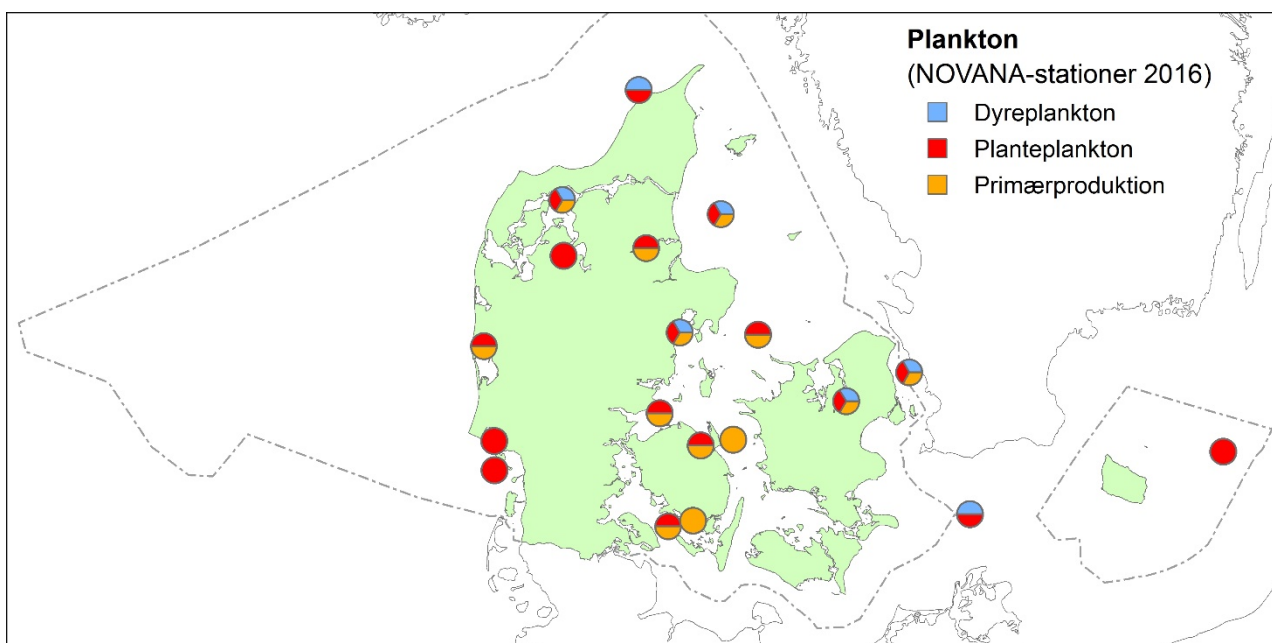
Figur 1.2. Prøvetagningsstationer for dyrep plankton, planteplankton og primærproduktion i 2016. Afgrænsning af de danske farvandsområder er angivet ved den stiplede linje (EEZ-grænse, Exclusive Economic Zone).
