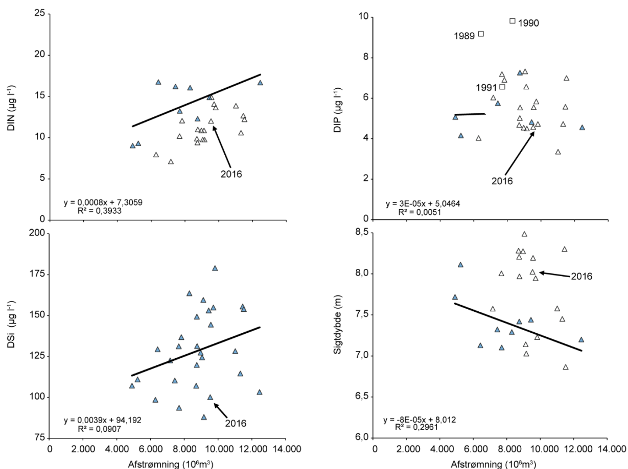
Figur B1.2. Årsmiddelkoncentrationer for DIN, DIP, DSI og sigtbybde i overfladevand for åbne havområder (0-10 m) mod afstrømning. Årene 1998-2016 er markeret med åbne trekanter for DIN, DIP og sigtbybde, og for DIP er årene 1989, 1990 og 1991 markeret med åbne firkanter.
