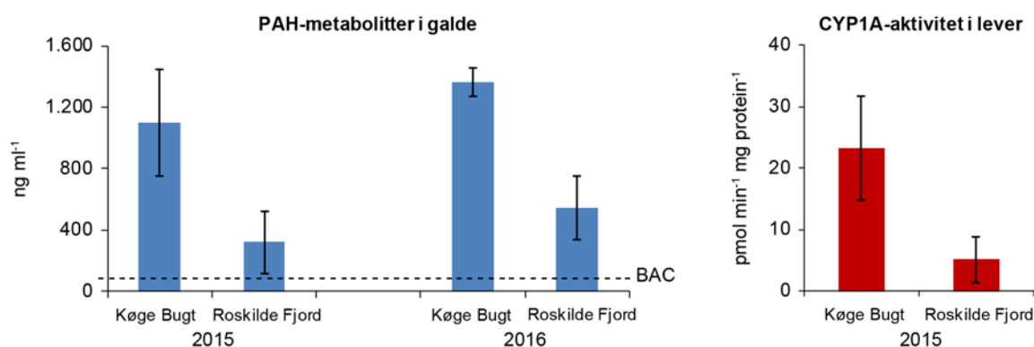
Figur 9.3. Niveaue af den PAH-specifikke effektindikator i ålekvar: PAH-metabolitter i galde undersøgt ved to stationer i 2015 og 2016 og CYP1A-aktivitet i 2015 (2016-analyser kasseret, se tekst).
