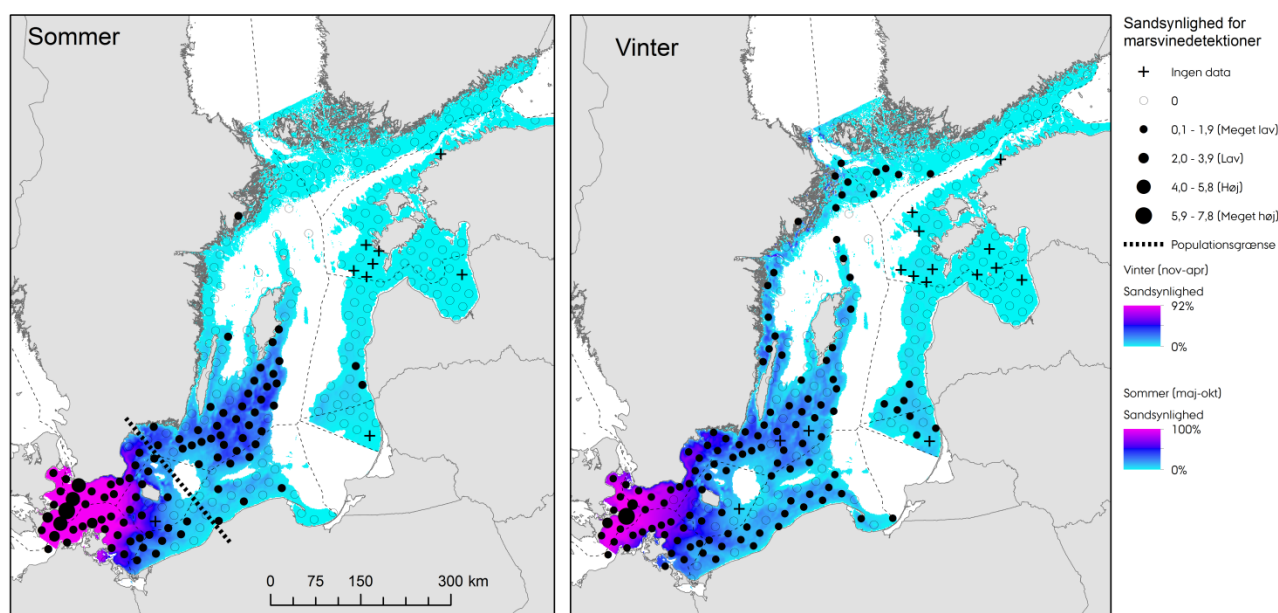
Figur 8.11. Model over sandsynlighed for marsvinetektioner om sommeren (maj-oktober) og vinteren (november-april). Lyseblå indikerer lav sandsynlighed og lilla indikerer høj sandsynlighed. Cirkler indikerer position for marsvinelyttestationer (C-POD) udlagt maj 2011-juni 2013 under SAMBAH-projektet. Størrelsen på udfyldte sorte cirkler indikerer antallet af marsvinetektioner, tomme cirkler indikerer ingen detektioner og krydser indikerer ingen data, hvilket oftest skyldtes mistet udstyr. Den stiplede linje viser den foreslåede sommer-populationsgrænse mellem Bælthavs- og Østersø-populationerne af marsvin.
