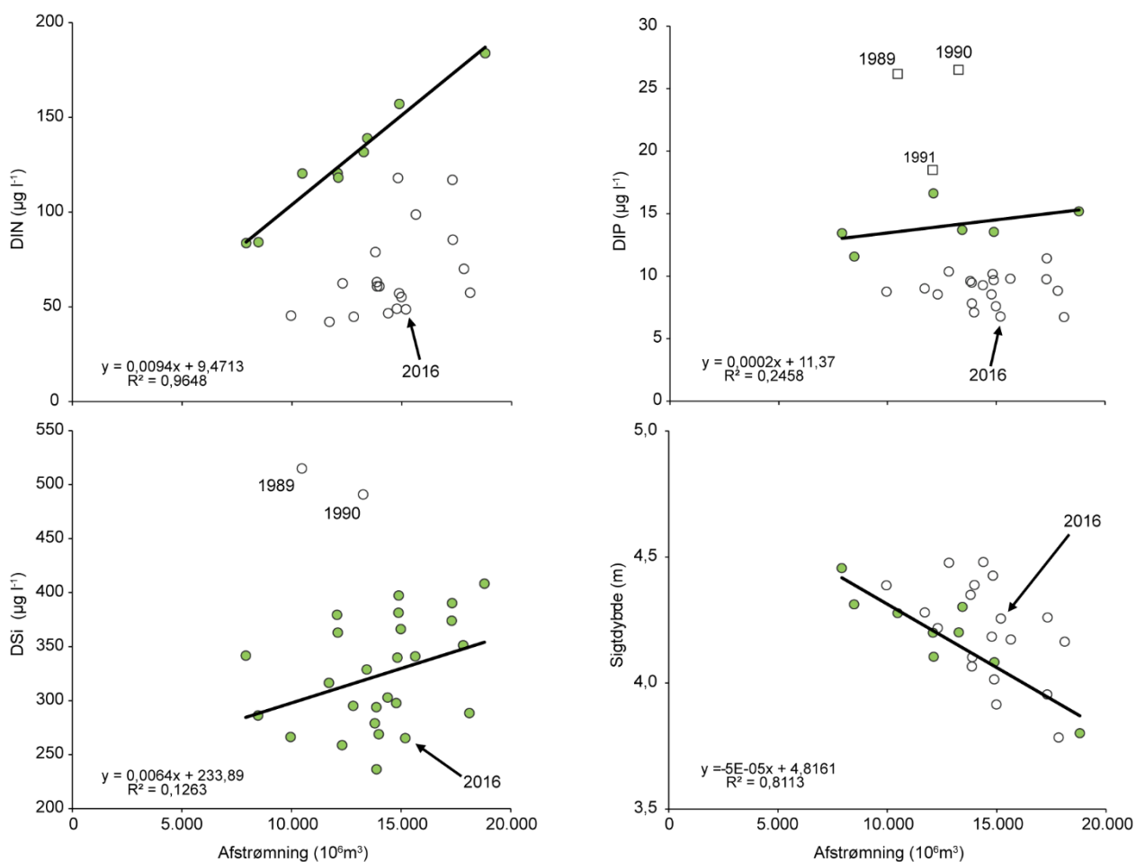
Figur B1.1. Årsmiddelkoncentrationer for DIN, DIP, DSi og sigtddybde i fjorde og kystvande mod afstrømning. Årene 1998-2016 er markeret med åbne cirkler for DIN, DIP og sigtddybde. For DIP er årene 1989-1991 markeret med åbne firkanter, og for DSi er årene 1989 og 1990 markeret med åbne cirkler.
