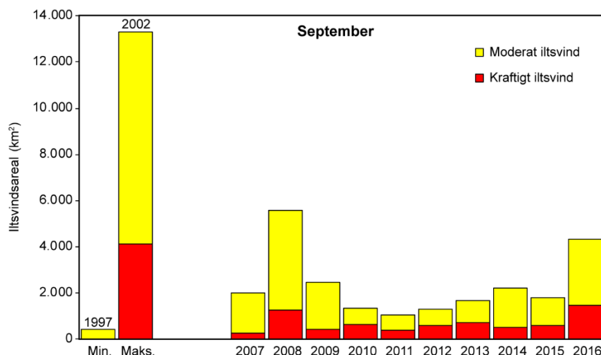
Figur 5.4. Udviklingen i arealet af moderat iltsvind ( 2\text{--}4 \text{ mg l}^{-1} ) og kraftigt iltsvind ( < 2 \text{ mg l}^{-1} ) i september i de indre danske farvande for perioden 2007-2016 samt den største og mindste registrerede arealudbredelse i overvågningsperioden 1989-2016. Til sammenligning har Fyn et areal på ca. 3.000 \text{ km}^2 og Sjælland et areal på ca. 7.000 \text{ km}^2 .
