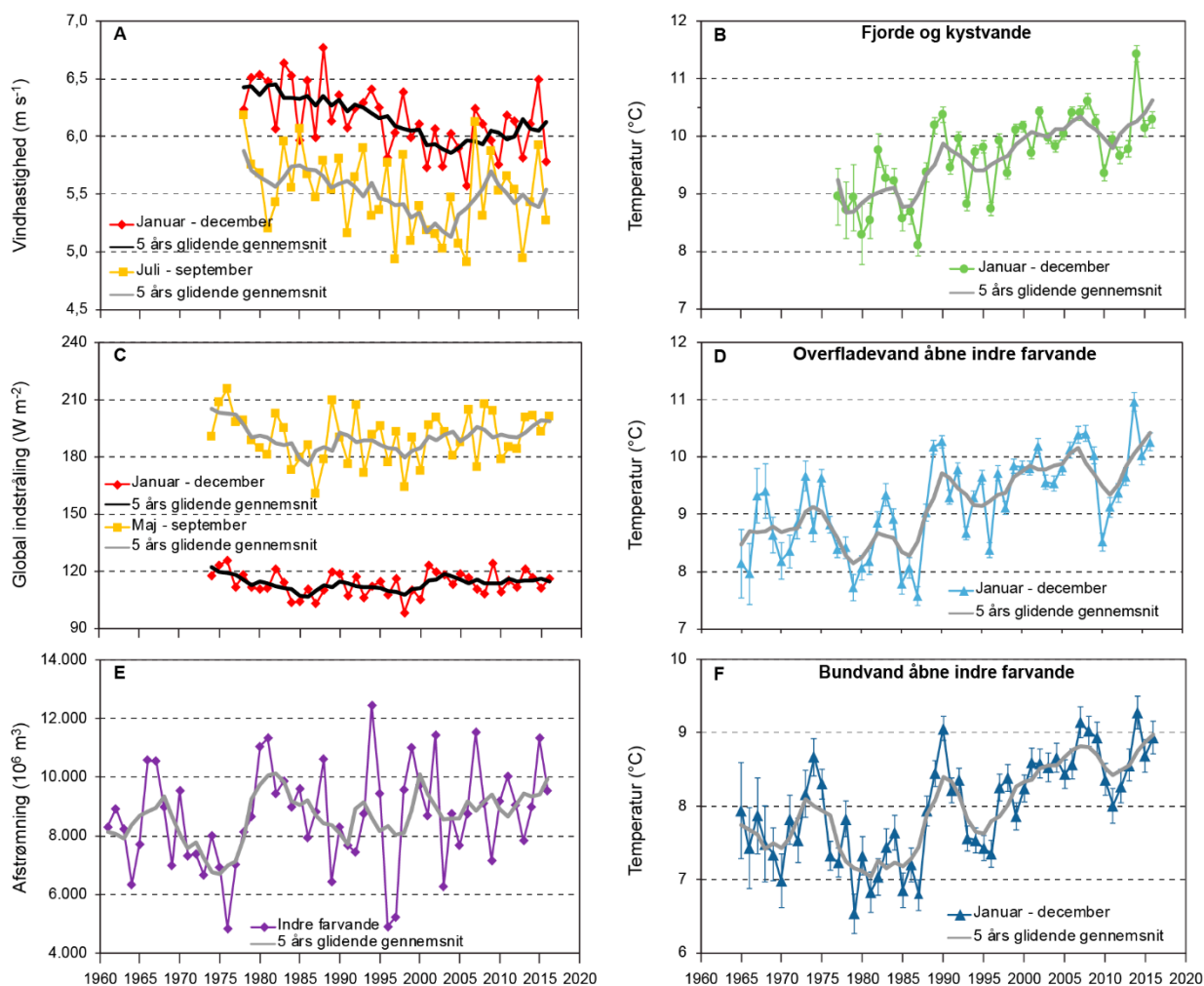
Figur 2.3. Tidslig udvikling for A) vindhastighed, B) vandtemperatur i fjorde og kystvande, C) indstråling, D) overfladevands-temperatur i de åbne indre farvande, E) afstrømning til de åbne indre farvande og F) bundvandstemperatur i de åbne indre farvande. Datakilder: Sund og Bælt Holding, DTU Vindenergi, H.C. Ørsted Instituttet, Landbohøjskolen (A og C); DCE og Miljøstyrelsen (B, D, E og F). Middeltemperaturer er angivet med 95 % konfidensgrænser.
