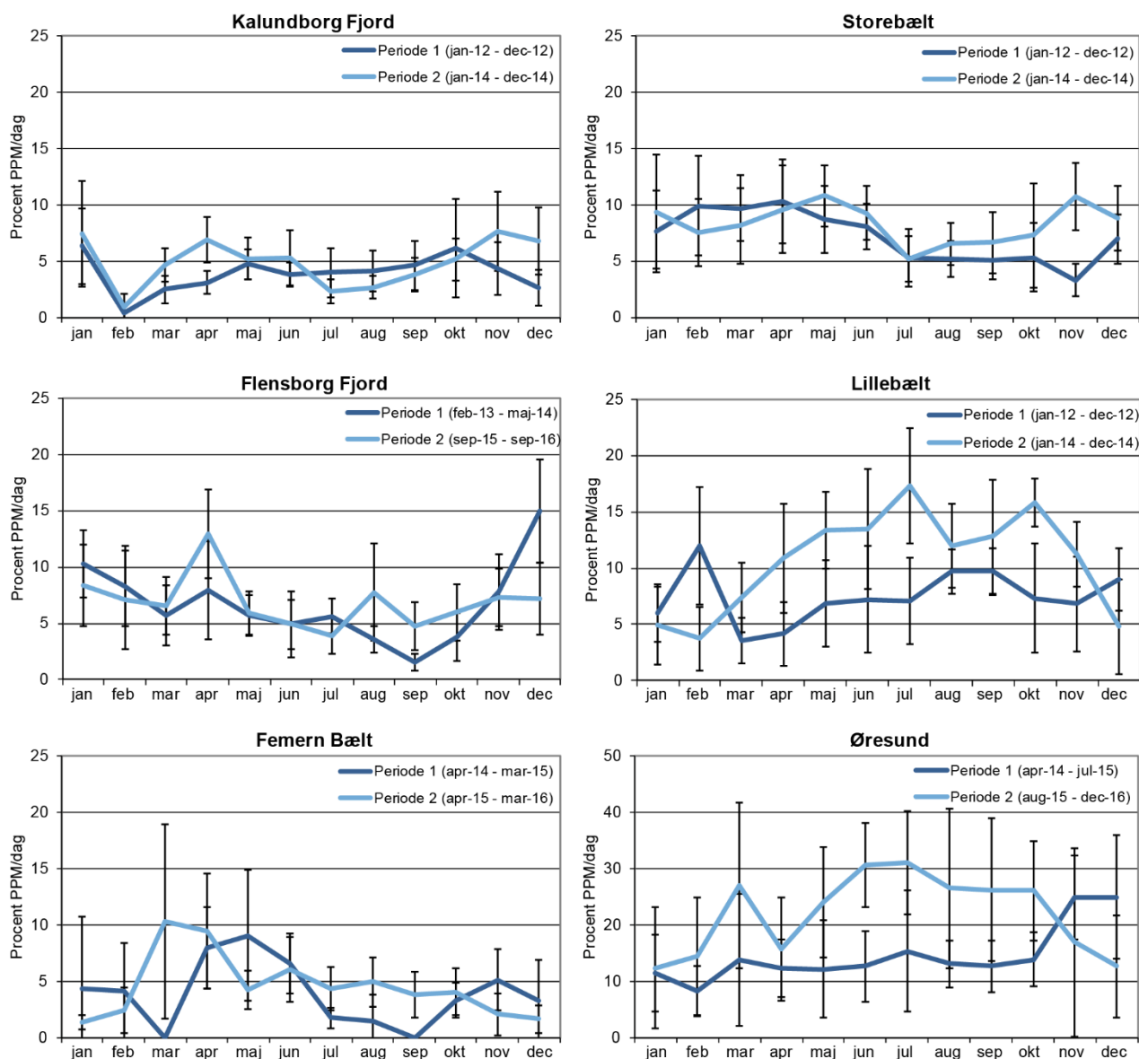
Figur 8.7. Gennemsnit af marsvinpositive minutter pr. døgn (PPM) i procent af døgnet fordelt på måneder og de to overvågningsperioder (figur 8.3) for de fem akustiske lytteposter anvendt i hver af de seks Natura 2000-områder i de indre danske farvande 2012-2016. Vertikale linjer indikerer standardafvigelse fra middelværdien. Bemærk at skalaen på y-aksen for grafen for Øresund er anderledes end de øvrige. Flensborg Fjord = Flensborg Fjord, Bredgrund og farvandet omkring Als, Storebælt = Centrale Storebælt og Vresen, Kalundborg Fjord = Røsnæs, Røsnæs Fjord og Kalundborg Fjord, Øresund = Gilleleje Flak og Tragten.
