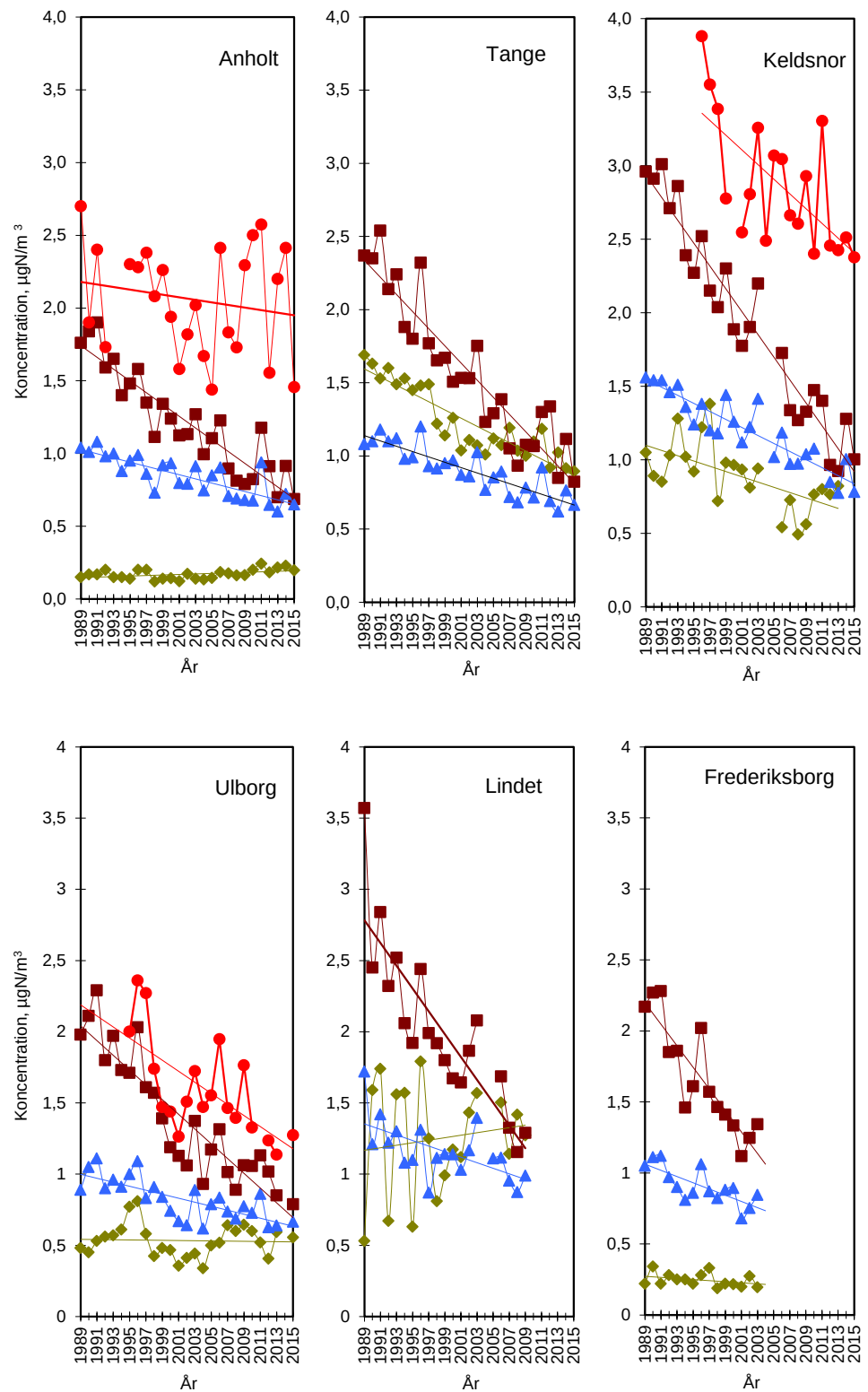
Figur A3. Årsmiddelkoncentrationer af kvælstofdioxid (rød), ammoniak (grøn), partikulært ammonium (brun), og partikulært nitrat (blå). Målingerne ved Lindet og Frederiksborg er ophørt i henholdsvis 2009 og 2003. Målingerne med filterpackopsamler ved Keldsnor er ophørt i 2009 og videreført med denuder fra 2010.
