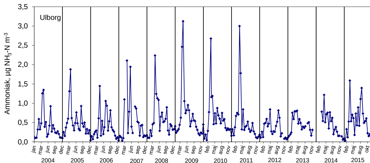
Figur 2.8. Koncentrationer af gasformig ammoniak målt på Ulborg i perioden 2004-2015. Målingerne er halvmånedsmiddelværdier (markeret med start for opsamlingsperiode). De manglende data for december 2013 til marts 2014 skyldes stormvejret, som ødelagde målestationen i december 2013.
