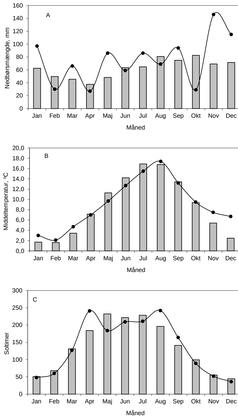
Figur 1.4. Månedlig nedbør (A); middellufttemperatur (B) og antal soltimer (C). Arealvægtede gennemsnit for Jylland og Øerne. Kurverne angiver resultater for 2015, mens søjlerne angiver middel for 1989-2014. Data er fra Cappelen og Jørgensen (2007) og DMI (2016).
