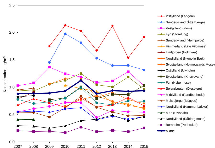
Figur 2.13. Årsmiddeldkoncentrationer af ammoniak i perioden fra 2007 til 2015 på en række naturlokaliteter fordelt over landet. Middel repræsenterer et vægtet middel af den gennemsnitlige udviklingstendens for målestationerne, som har været aktive fra 2007-2015.
