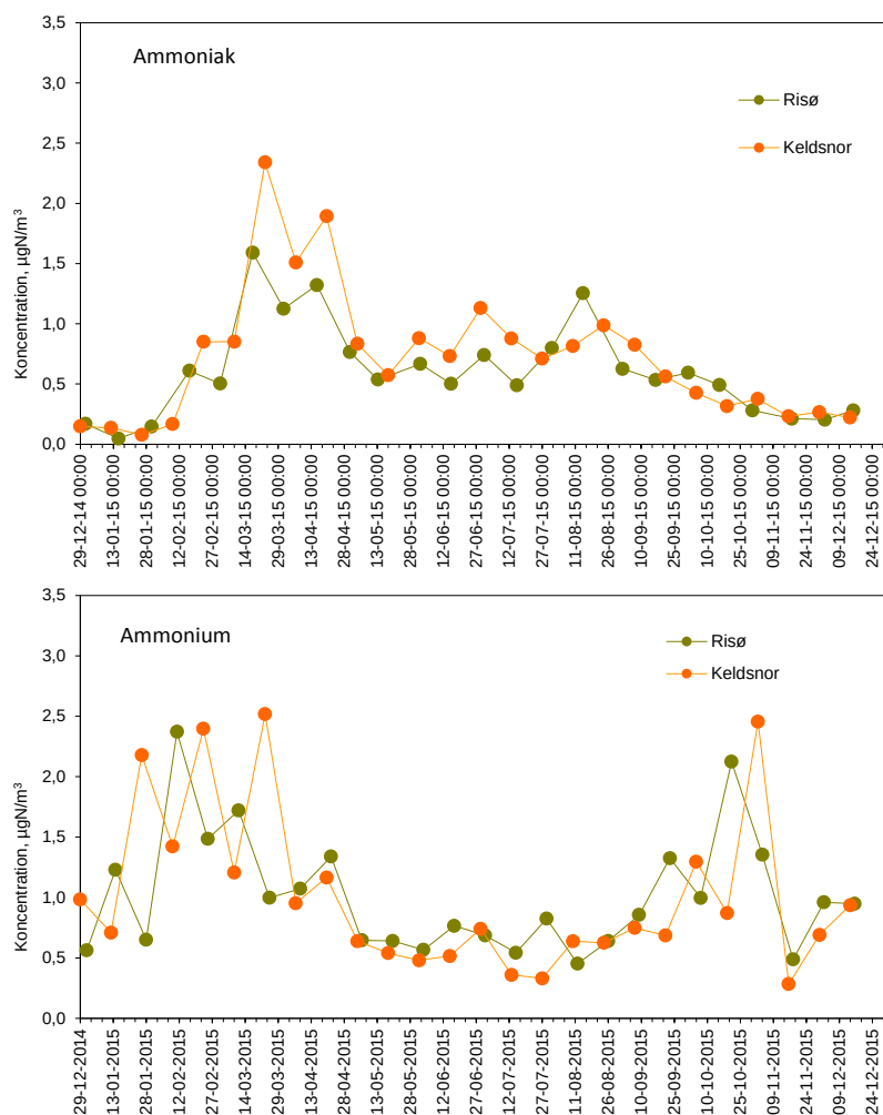
Figur 2.7. Koncentration af gasformig ammoniak ( \text{NH}_3 ) og partikulært ammonium ( \text{NH}_4^+ ) målt på Keldsnor og Risø i 2015. Målingerne fra Risø ( \text{NH}_3 – passiv opsamler; \text{NH}_4 - filter-pack) er halvmånedsmiddelværdier (markeret med start for opsamlingsperiode), mens målingerne fra Keldsnor (denuder) er ugemiddelværdier, som for sammenlignelighedens skyld er blevet midlet til to-ugersmiddelværdier.
