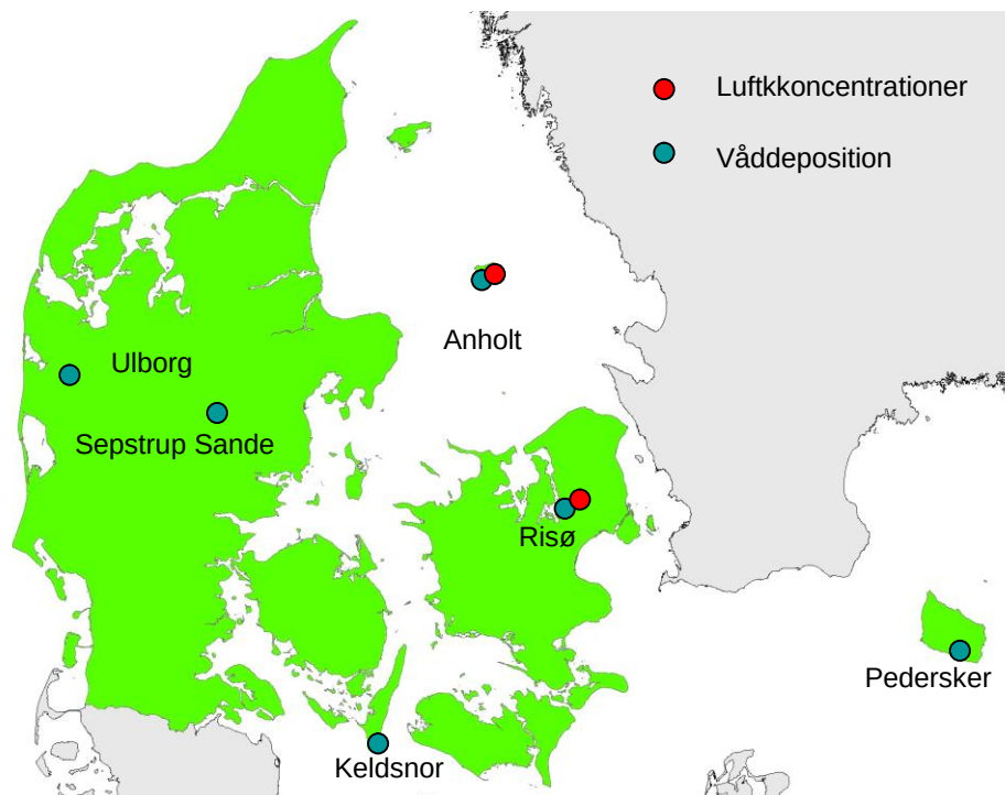
Figur 4.1. Målestationer hvor der måles luftkoncentrationer og våddeposition af tungmetaller i Danmark i 2015.
