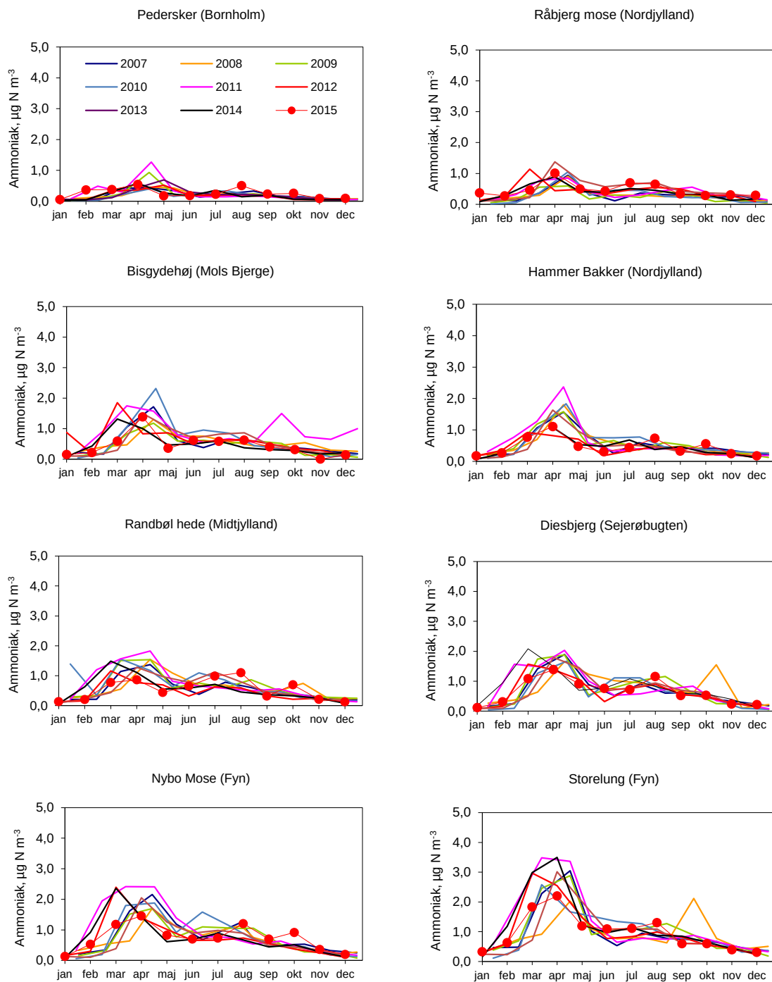
Figur 2.11. Koncentrationer af ammoniak på en række stationer i årene 2007-2015. Målingerne er månedsmiddel og markeret ved start, som er d. 15. i måneden i perioden fra 2007-2011 og d. 1. i måneden i 2012-2015.
