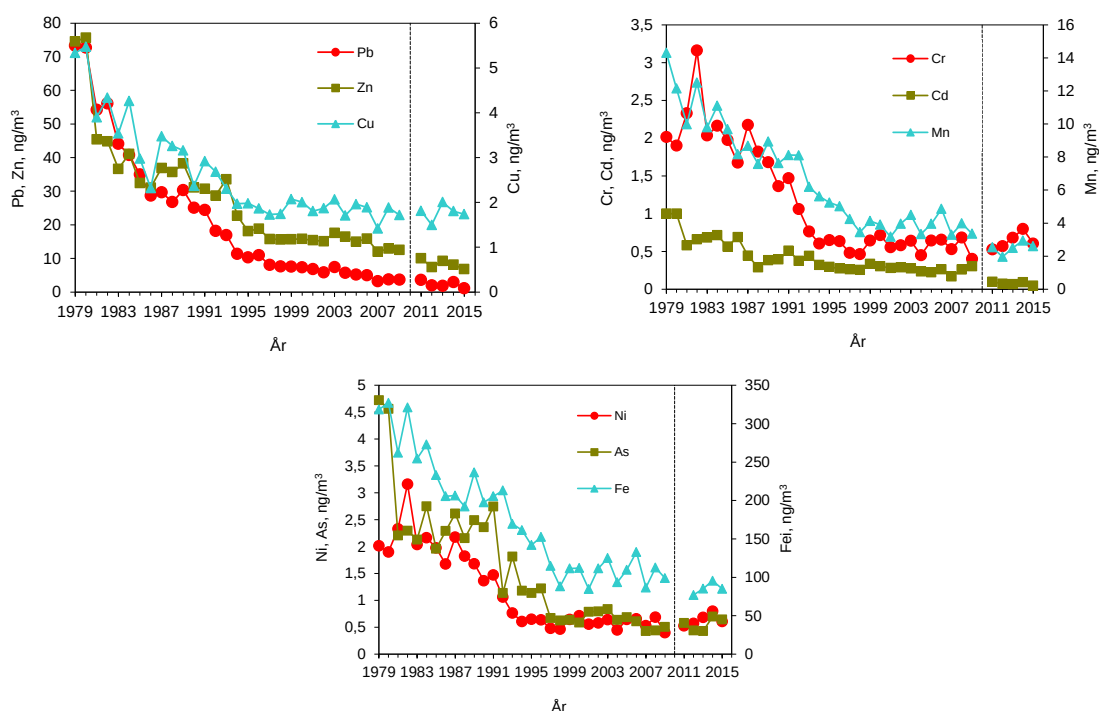
Figur 4.3. Udvikling af koncentrationer i luften af en række tungmetaller siden 1979. Kurverne repræsenterer gennemsnit af målinger ved Keldsnor og Tange i perioden før 2010, mens 2011-2015 er beregnet som gennemsnit for Anholt og Risø. Den sorte stiplede linje indikerer dette skift i målestationerne.
