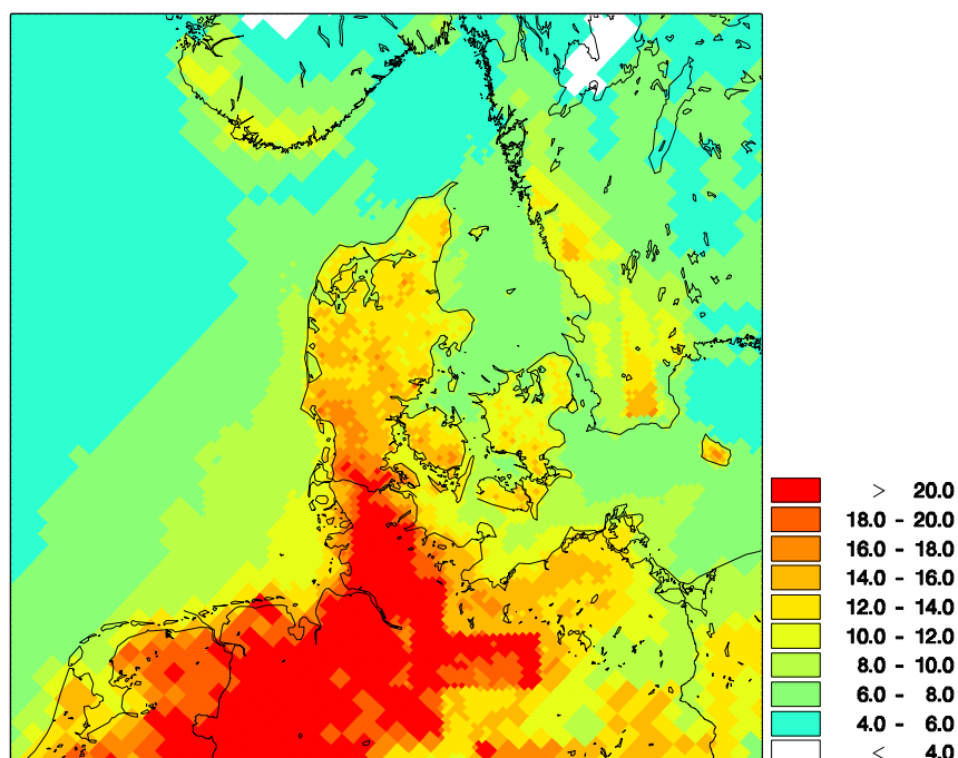
Figur 2.2. Den samlede deposition af kvælstofforbindelser beregnet for 2015. Depositionen angiver en middelværdi for felterne. For felter med både vand- og landoverflade vises altså en middeldeposition for de to typer af overflade. Depositionen er givet i kg N/ha. Gitterfelterne er på 6 km x 6 km undtagen for den yderste del af domænet, hvor gitterfelterne er på 17 km x 17 km.
