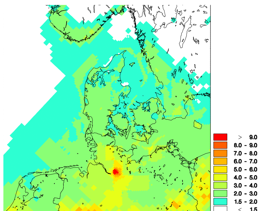
Figur 3.2. Den samlede antropogene deposition af svovlforbindelser beregnet for 2015. Depositionen angiver en middelværdi for felterne; for felter med både vand- og landoverflade vises altså en middeldeposition for de to typer af overflade. Depositionen er givet i kg S/ha. Gitterfelterne er på 6 km x 6 km undtagen for den yderste del af domænet, hvor gitterfelterne er på 17 km x 17 km. Den højere deposition i farvandsområderne skyldes skibstrafik. Den højeste deposition på land ses i Fredericia og skyldes store udledninger fra raffinaderiet.
