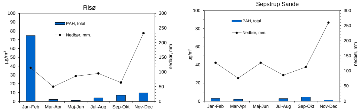
Figur 6.5. Samlet våddeposition af PAH i 2015 målt over 2-måneders perioder, \mu\text{g}/\text{m}^2 . Kurven angiver nedbørsmængde i de tilsvarende perioder i mm.
