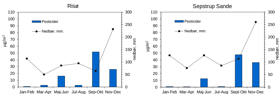
Figur 6.1. Våddepositionen, \mu\text{g}/\text{m}^2 , af de fundne pesticider og nedbrydningsprodukter i 2015 målt over 2-måneders perioder på Risø og Sepstrup Sande. Kurven angiver nedbørsmængde i den tilsvarende periode i mm.
