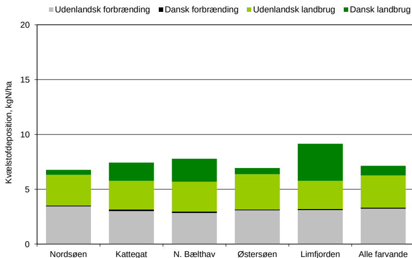
Figur 2.3. Gennemsnitlig kvælstofdeposition i 2015 til udvalgte danske farvandsområder og Limfjorden opdelt på danske og udenlandske kilder samt opdelt på emissioner fra forbrændingsprocesser og landbrugsproduktion.
