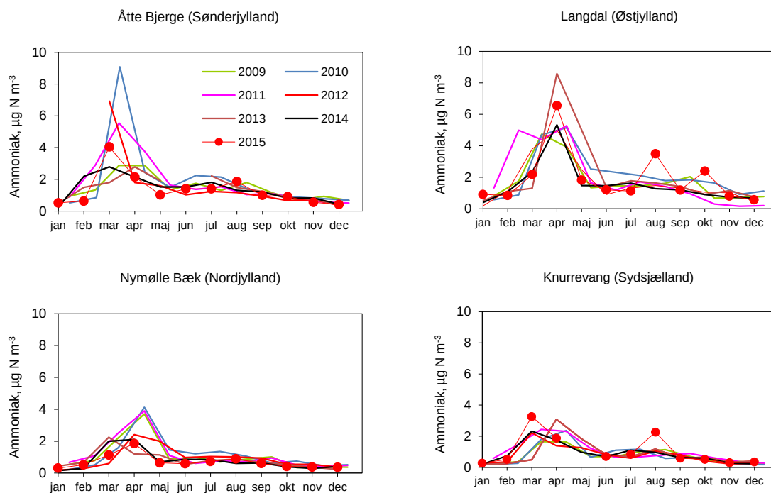
Figur 2.12. Koncentrationer af ammoniak på fire overdrevsstationer beliggende tæt ved landbrug i årene 2009-2015. Målingerne er månedsmiddelværdier og markeret ved start, som er d. 15. i måneden i perioden fra 2007-2011 og d. 1. i måneden i 2012-2015.
