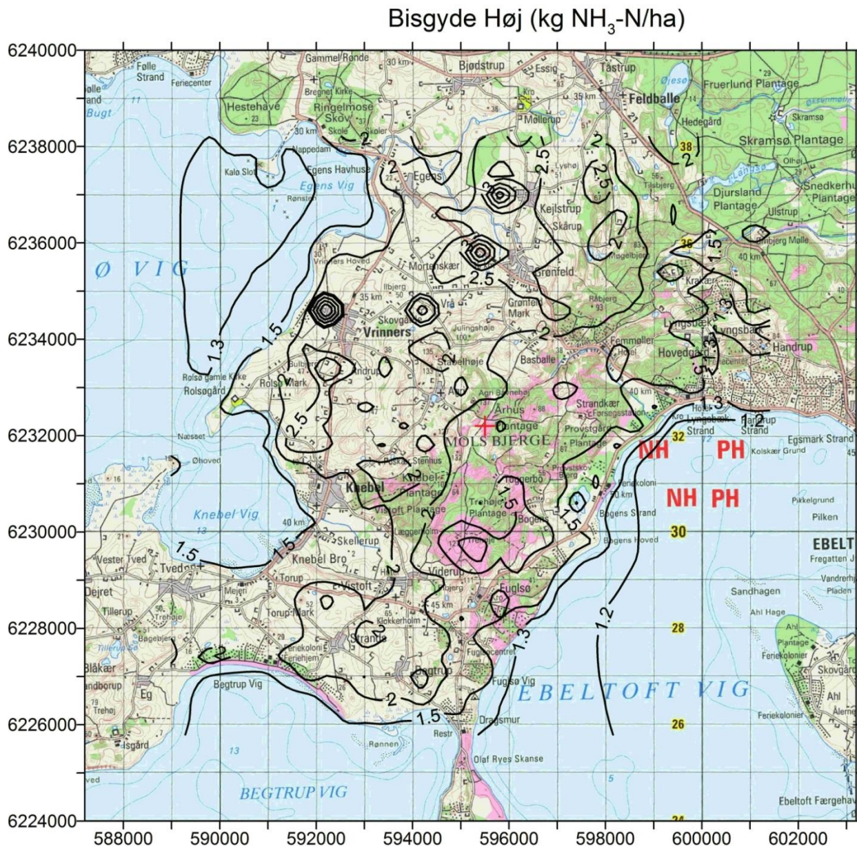
Figur 2.14 Den beregnede geografiske variation af tørdeponeret ammoniak i 2015 i et 16 km x 16 km område i Mols Bjerge. Isolinjerne angiver depositionerne 1,1; 1,2; 1,3; 1,5; 2; 2,5; 3; 4; 5 og 6 kg N/ha/år. Kurverne er ikke ført helt til kanten af kortområdet, idet usikkerheden her er større. Beregningen af depositionen er foretaget på basis af et net af felter på 400m x 400m. Det røde kryds midt i kortet angiver punktet, hvor depositionen til Bisgyde Høj (Overdrev, sure (6230)) i tabel 2.4 er beregnet. Værdierne på akserne angiver placering af området i UTM 32 nettet (m Øst og m Nord).
