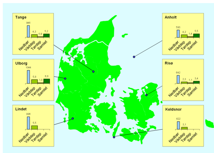
Figur 3.1. Svovldeposition (kg S/ha) og nedbørsmængde (mm) ved målestationerne i 2015. Svovldepositionen er beregnet til den gennemsnitlige landoverflade omkring målestationen. Nedbørsmængden er angivet i mm og depositionen er angivet i kgS/ha. Resultaterne fra Tange er baseret på kombination af målingerne ved Tange og Sepstrup Sande (se Figur 1.1). Der bliver ikke målt tørdeposition ved Keldsnor og Lindet.
