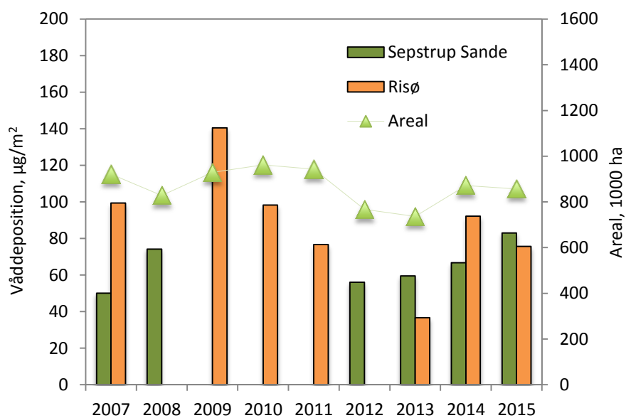
Figur 6.2. Årlig våddeposition ( \mu\text{g}/\text{m}^2 ) af prosulfocarb i Sepstrup Sande og Risø (2007-2015), samt udviklingstendens for areal med vintersæd. Kun de år, hvor der foreligger resultater for prøveopsamlinger i september-oktober og november-december, er medtaget i figuren. Huller i tidsserien skyldes tekniske problemer med prøveopsamlingen (fx nedbrud på opsamler, frostsprængning af opsamlingsflasker) i perioden fra september til december.
