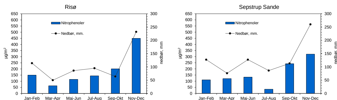
Figur 6.4. Samlet våddeposition af nitrophenoler i 2015 målt over 2-måneders perioder, \mu\text{g}/\text{m}^2 . Kurven angiver nedbørsmængde i de tilsvarende perioder i mm.
