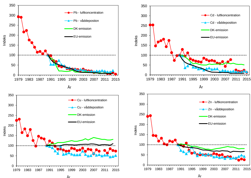
Figur 4.4. Målinger af våddeposition og partikelkoncentration i luften sammenlignet med emissioner fra Danmark og EU-landene (EMEP 2016). Alle resultater er normeret til 100 i 1990. Før 2010 er luftkoncentrationer beregnet som gennemsnit af Keldsnor og Tange og efter 2010 er de beregnet ud fra gennemsnit af Anholt og Risø.
