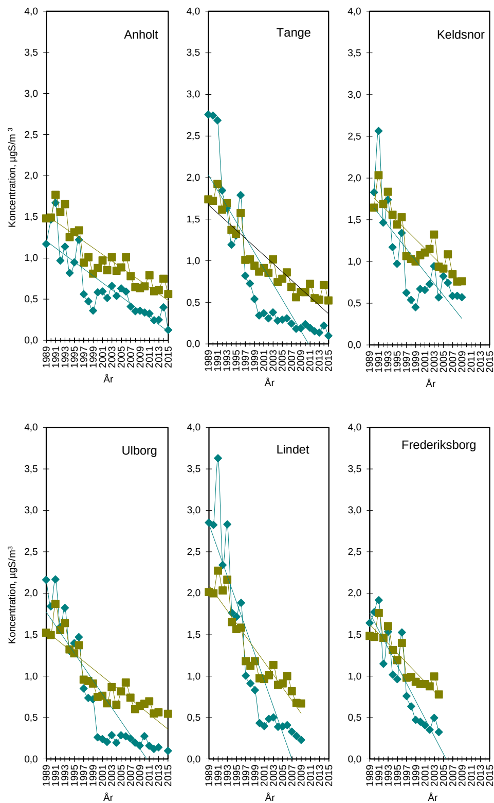
Figur A4. Årsmiddelkoncentrationer af svovldioxid (blå) og partikulært sulfat (grøn). Målingerne ved Keldsnor, Lindet og Frederiksborg er ophørt i 2010, 2009 og 2004.
