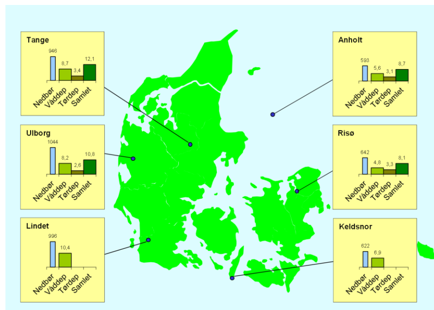
Figur 2.1. Kvælstofdeposition (kgN/ha) og nedbørsmængde (mm) ved målestationerne i 2015. Figuren angiver deposition til den gennemsnitlige landoverflade omkring målestationerne. Resultaterne fra Tange er baseret på kombination af målingerne ved Tange og Sepstrup Sande (se Figur 1.1). Grundet revision af programmet indgår tørdepositionen ikke længere ved Lindet og Keldsnor.
