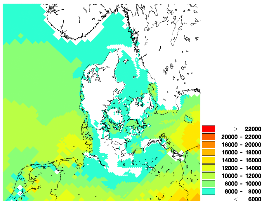
Figur 5.4. AOT40 beregnet med DEHM i henhold til EU's luftkvalitetsdirektiv. Enheden er \mu\text{g}\cdot\text{m}^{-3}\cdot\text{timer} , hvilket ganges med 0,5 for at komme til ppb-timer.
