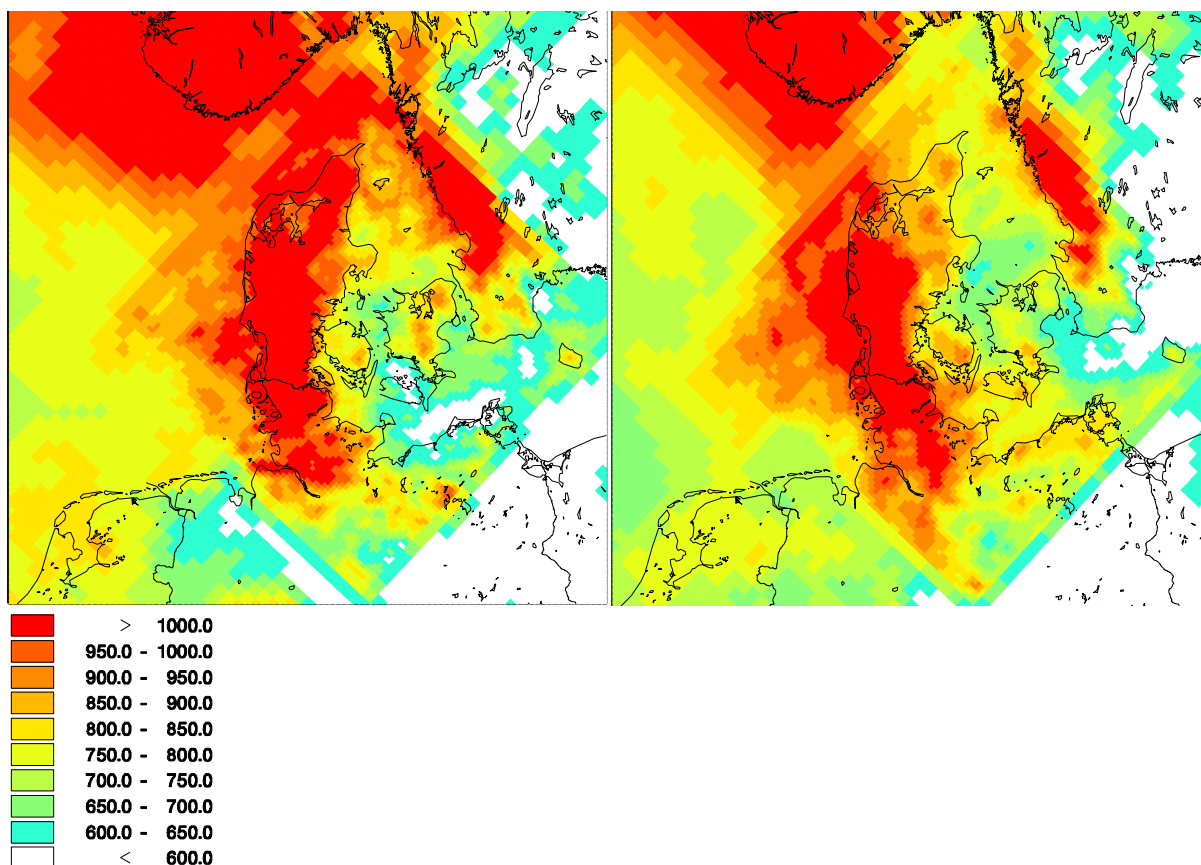
Figur 1.5. Nedbørsmængder beregnet med den meteorologiske model MM5 for 2014 (venstre) og 2015 (højre). Nedbøren er angivet i mm. Nedbørsmængderne er primært beregnet af hensyn til modelberegningerne af luftkvalitet og deposition, men giver også et overblik over de geografiske variationer i nedbøren.
