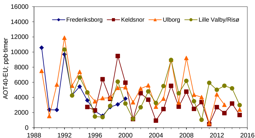
Figur 5.3. AOT40-værdier for vegetation (enheden er ppb-timer) for vegetation beregnet i henhold til EU's luftkvalitetsdirektiv (EC 2008) for målestationerne Keldsnor, Frederiksborg, Ulborg og Lille Valby/Risø. AOT40 er beregnet på basis af ozonmålinger i maj til juli fra kl. 8.00 til 20.00.
