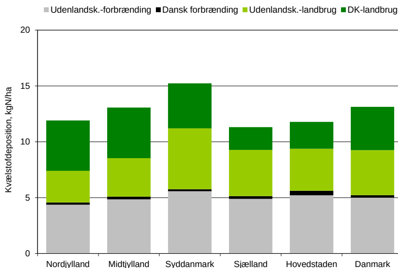
Figur 2.4. Gennemsnitlig kvælstofdeposition i 2015 til de nye regioner og i gennemsnit for hele landet (Danmark) opdelt på danske og udenlandske kilder samt opdelt på emissioner fra forbrændingsprocesser og landbrugsproduktion.
