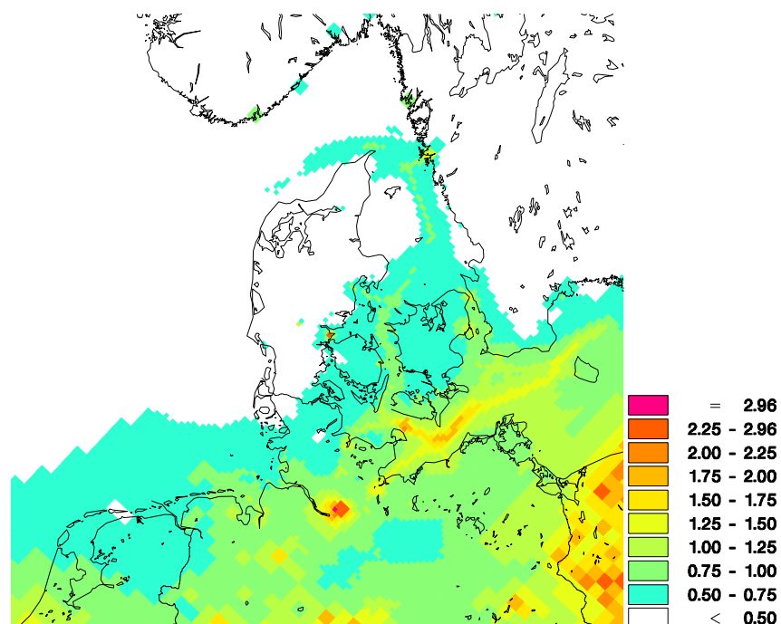
Figur 3.4. Vintermiddeldkoncentrationer (1. oktober – 31. marts) af SO 2 i 2015 beregnet med luftforureningsmodellen DEHM. Enheden er µg SO 2 /m 3 . Den højeste koncentration ses i Fredericia og skyldes udledninger fra raffinaderiet.
