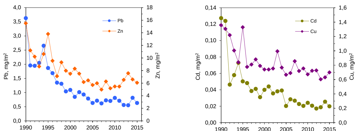
Figur 4.2. Tidsudvikling i årlig våddeposition over en 26-årig periode af Zn og Pb (venstre figur) og Cu og Cd (højre figur). Enhed er mg metal per m^2 , hvilket svarer til kg/km^2 .
