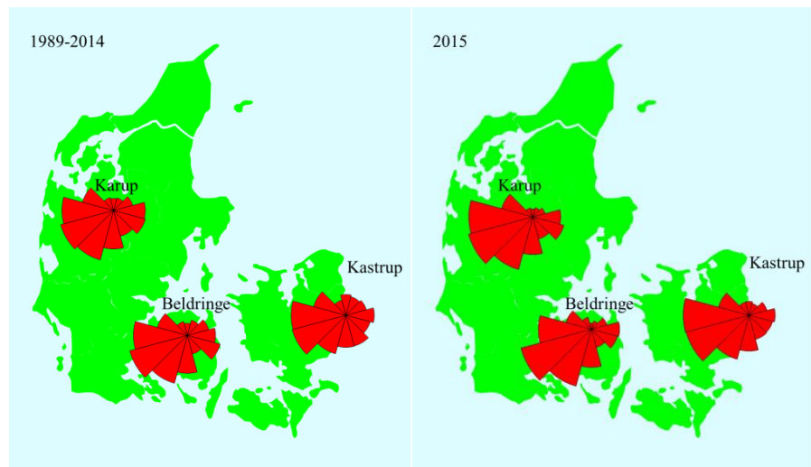
Figur 1.3. Vindroser for Karup, Beldringe, og Kastrup. Til venstre vises gennemsnit for perioden 1989-2014, mens der til højre vises gennemsnit for 2015. Måling af vindretning er udført af Danmarks Meteorologiske Institut (DMI).
