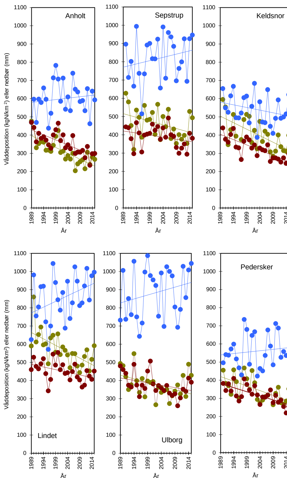
Figur A1. Årlig våddeposition (kgN/km 2 ) af ammonium (grøn) og nitrat (brun) siden 1989 samt nedbørsmængde (blå, mm). KgN/km 2 omregnes til kgN/ha ved at dividere med 100.
