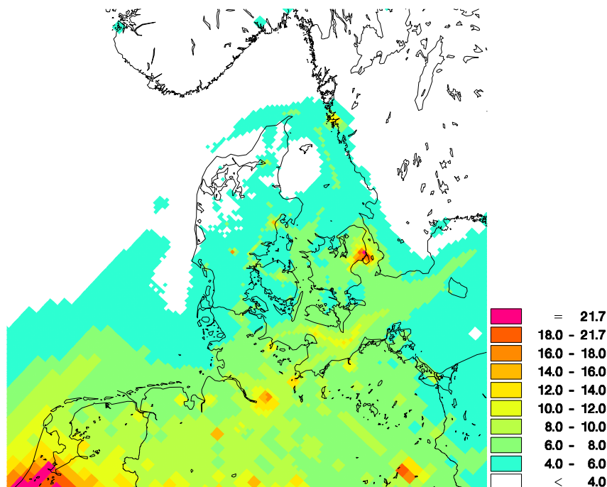
Figur 2.6. Årsmiddelkoncentrationer af NO x i 2015 beregnet med luftforureningsmodellen DEHM. Enhed er koncentrationen af NO x beregnet som NO 2 (µg NO 2 /m 3 ).
