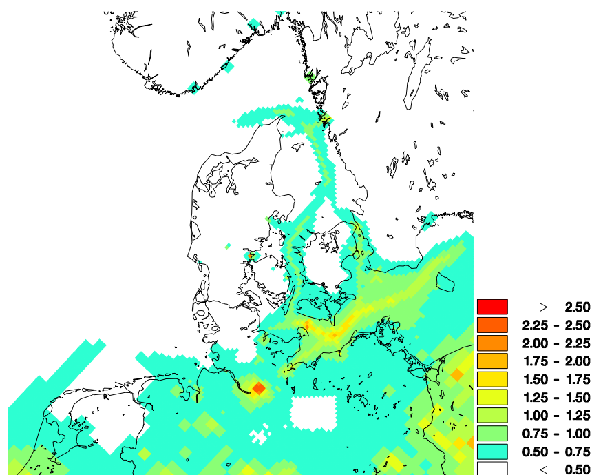
Figur 3.3. Årsmiddelkoncentrationer af SO 2 i 2015 beregnet med luftforureningsmodellen DEHM. Enheden er µg SO 2 /m 3 . Den højeste koncentration ses i Fredericia og skyldes udledninger fra raffinaderiet.
