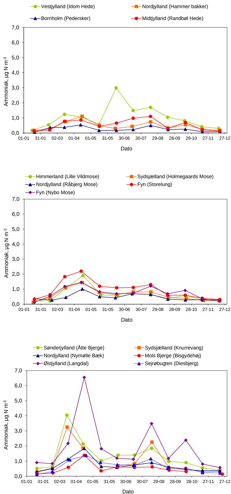
Figur 2.10. Koncentrationer af gasformig ammoniak i 2015 på en række naturlokaliteter fordelt over landet. Målingerne er månedsmiddelværdier markeret ved midten af opsamlingsperioden. Bemærk de forskellige y-akseinddelinger. Øverst: hede (Idom Hede: månedsmiddelværdierne er midlet fra målinger på halvmånedsbasis). Midt: højmoser og hængesæk. Nederst: sure overdrev.
