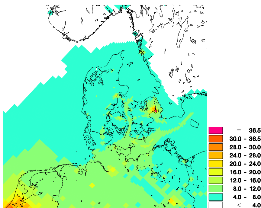
Figur 2.6. Årsmiddelt koncentrationer af NO x i 2014 beregnet med luftforureningsmodellen DEHM. Enhed er µg NO x /m 3 .
