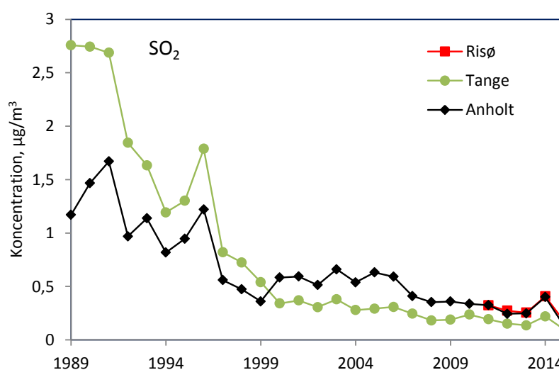
Figur 8.2. Årsmiddelmålinger af svovldioxid angivet som \mu\text{g S/m}^3 . Data for 2015 dækker kun perioden fra januar til maj.
