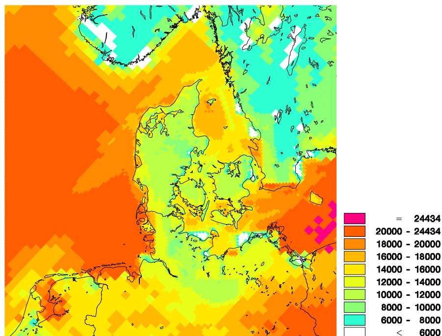
Figur 6.4. AOT40 beregnet med DEHM i henhold til EU's luftkvalitetsdirektiv. Enheden er \mu\text{g}\cdot\text{m}^{-3}\cdot\text{timer} , hvilket ganges med 0,5 for at komme til ppb-timer.
