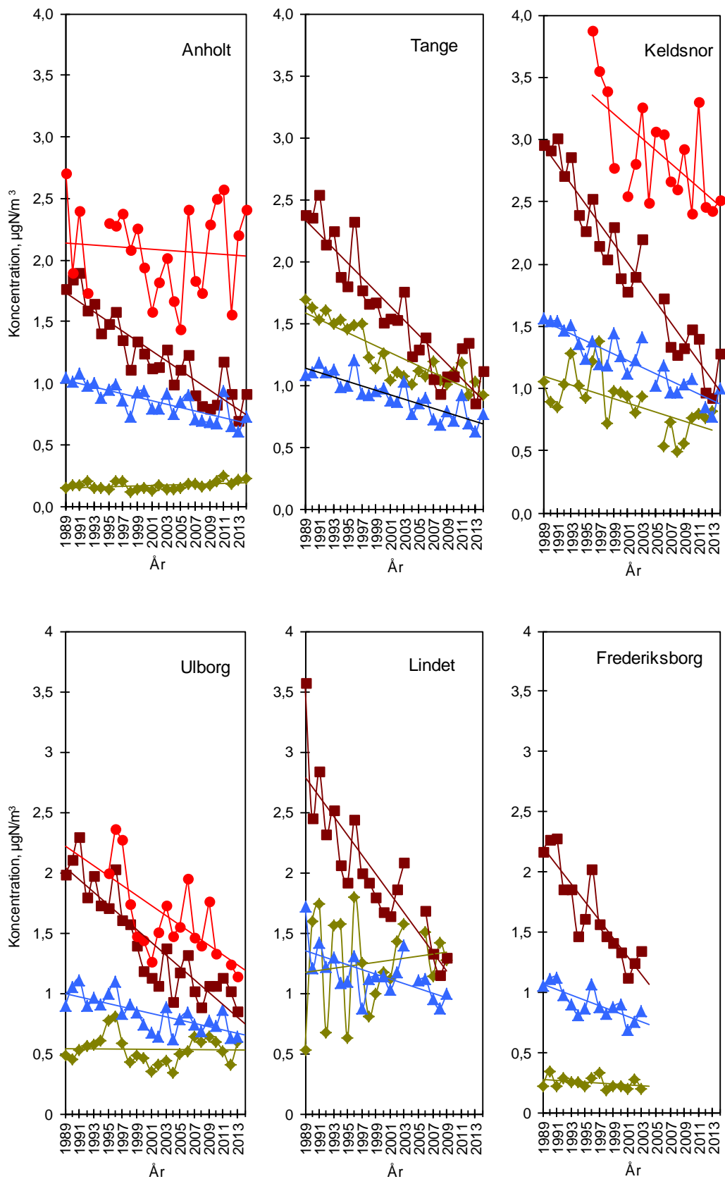
Figur A3. Årsmiddeldkoncentrationer af kvælstofdioxid (rød), ammoniak (grøn), partikulært ammonium (brun), og partikulært nitrat (blå). Målingerne ved Lindet og Frederiksborg er ophørt i henholdsvis 2009 og 2003. Målingerne med filterpakkopsamler ved Keldsnor er ophørt i 2009.
