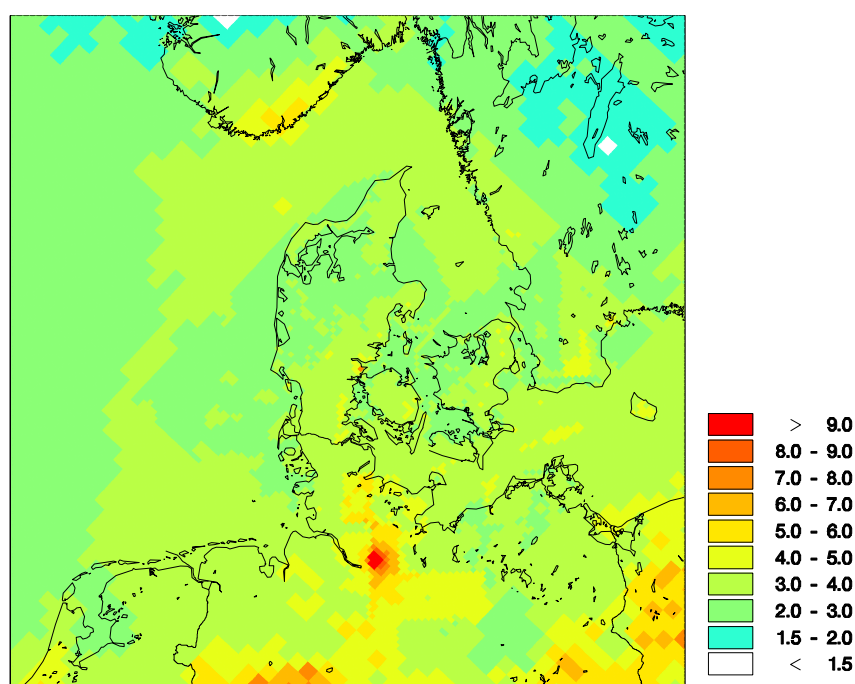
Figur 4.2. Den samlede antropogene deposition af svovlforbindelser beregnet for 2014. Depositionen angiver en middelværdi for felterne; for felter med både vand- og landoverflade vises altså en middeldeposition for de to typer af overflade. Depositionen er givet i kg S/ha. Gitterfelterne er på 6 km x 6 km undtagen for den yderste del af domænet, hvor gitterfelterne er på 17 km x 17 km. Den højere deposition i farvandsområderne skyldes skibstrafik. Den højeste deposition på land ses i Fredericia og skyldes store udledninger fra raffinaderiet.
