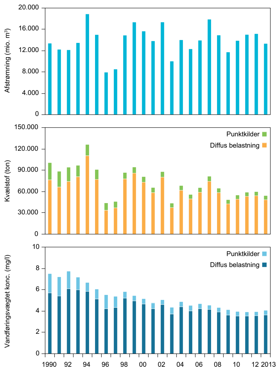
Figur 2.1. Udvikling i ferskvands-afstrømning (øverst), kvælstoftilførsel (midterst) og vandføringsvægtet kvælstofkoncentration i det afstrømmende vand til havet omkring Danmark (nederst) 1990-2013. Kvælstoftilførslen er fordelt på diffuse kilder (inkl. spildevand fra spredt bebyggelse) og spildevand fra punktkilder (Wiberg-Larsen et al. 2015).
