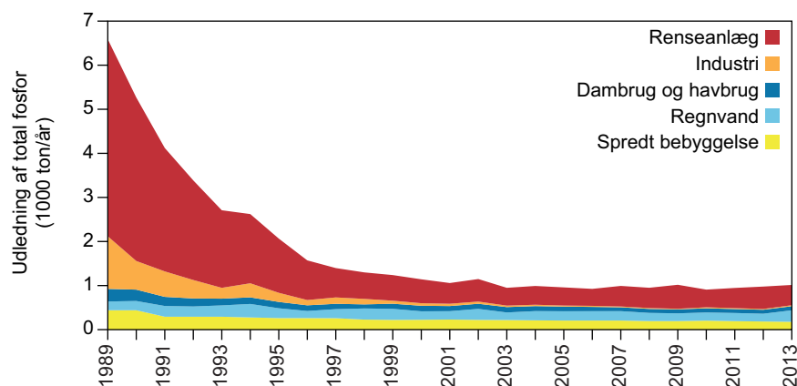
Figur 3.2. Udviklingen i de årligt udledte mængder af fosfor opdelt på forskellige punktkilder (Naturstyrelsen 2015).
