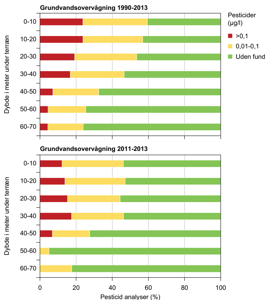
Figur 6.8. Dybdemæssig fordeling af hyppigheder af pesticidfund i grundvandsovervågningen i 1990-2013 og i 2011-2013. Datagrundlaget under 50 m.u.t. er begrænset for perioden 2011-2013. (Thorling et al. 2015).
