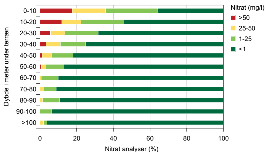
Figur 6.4. Fordeling af nitrat-indholdet i 2013 efter indtagedybde under terræn i land- og grundvandsovervågning, grundvand i indvindingsboringer og 'Andre boringer' (undersøgelingsboringer, pejleboringer, private boringer og brønde, afværgeboringer, lukkede vandværker m.v.) (Thorling et al. 2015).
