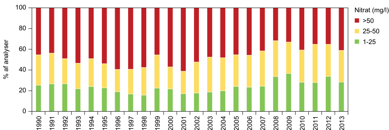
Figur 6.3. Fordeling af nitratindehold i perioden 1990-2013 i grundvand i iltzonen (med ilt > 1 mg/l). Den enkelte søjle repræsenterer grundvand fra flere indtag med forskellige aldre (Thorling et al. 2015).
