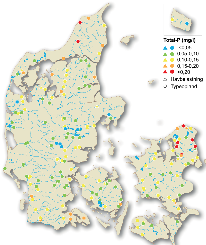
Figur 7.5. Koncentrationen af total fosfor i vandløb i 2013. Vandføringsvægtede årsmiddelværdier (Wiberg-Larsen et al. 2015).
