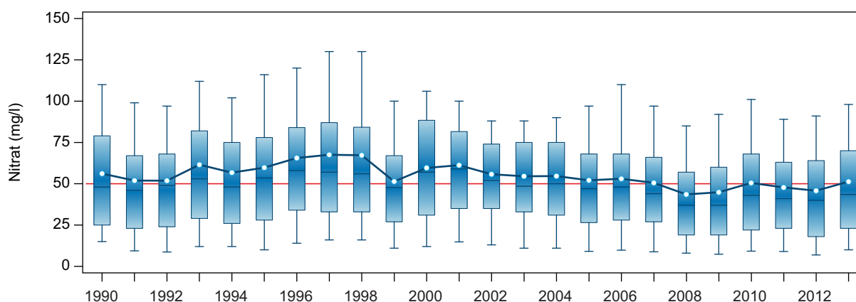
Figur 6.5. Udviklingen i nitratindhold i iltzonen i grundvand i perioden 1990-2013. Kurven i boksen forbinder medianværdierne. Desuden er vist 75 % og 25 % fraktiler i minimums og maksimumsværdier af analyseresultater det enkelte år (top og bund af boks), samt 90 % og 10 % fraktiler. Den orange linje viser kravværdien for nitrat i drikkevand og grundvand på 50 mg/l (Thorling et al. 2015).
