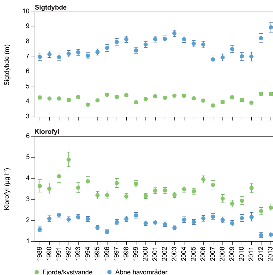
Figur 9.4. Udviklingen af årlige gennemsnitlige værdier for fjorde og kystnære områder og for de indre åbne farvande for sigtgybde og klorofylkoncentration (Hansen (red.) 2015).
