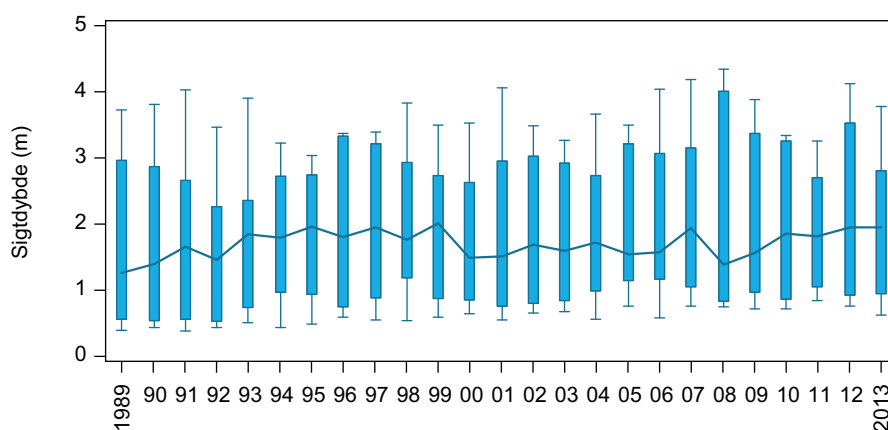
Figur 8.3. Udviklingen i sigtdybde (sommergenomsnit) i de 15 søer, der har været overvåget siden 1989. Søjlerne viser 10, 25, 75 og 90 % fraktiler. Linjen viser medianværdien (Bjerring et al. 2015).
