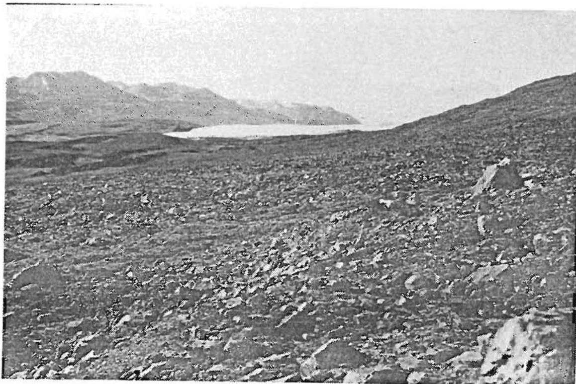
Fig. 2.8. Fjeldmark i stenet område ved Frigg Fjord, Peary Land. Foto: C. Bay.
