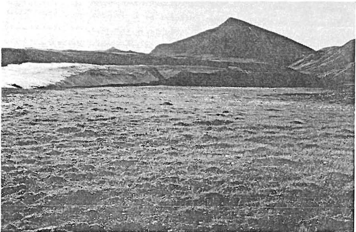
Fig. 2.15. Frodig vegetationsmosaik med kær og sneleje. Brainard Sund, Nansen Land. Foto: C. Bay.
