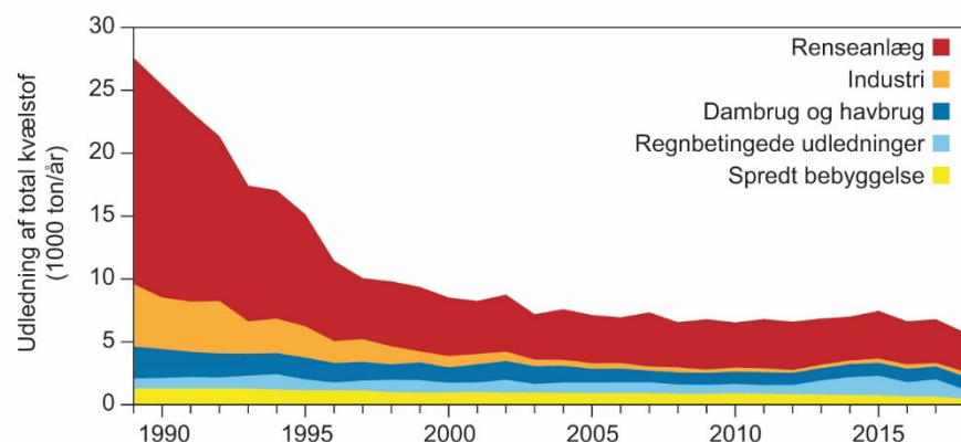
Figur 1.5. Udvikling i udledning af kvælstof fra forskellige typer punktkilder (Miljøstyrelsen 2019). Miljøstyrelsen finder ikke anledning til at udføre korrektioner på data grundet analysefejl (se indledning kap. 1).
