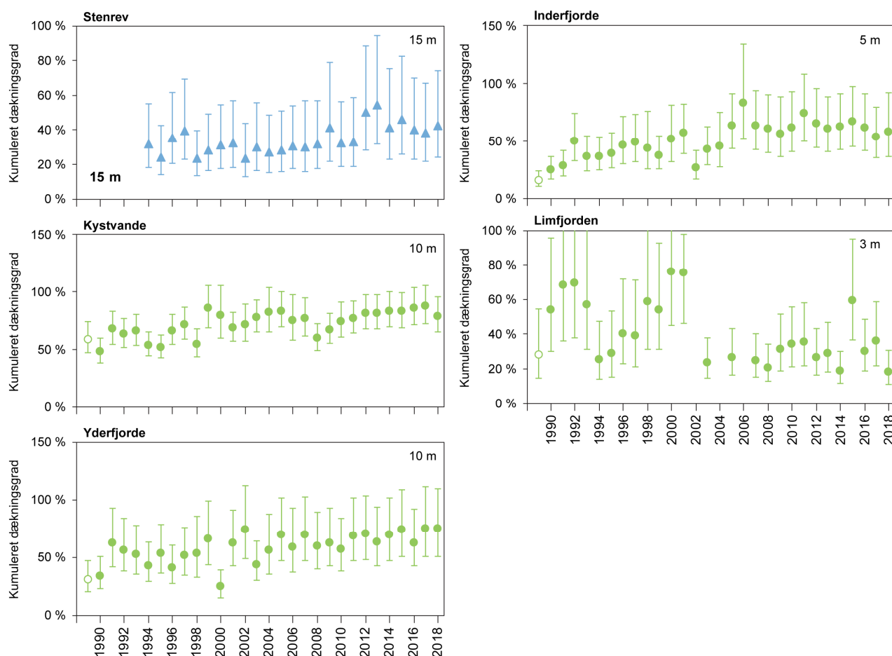
Figur 8.4. Makroalgerne kumulerede dækningsgrad i perioden 1989-2018 for stennrev i åbne farvande og på sten i kystvande, yder- og inderfjorde samt i Limfjorden. Data fra 1989 og for stennrev også fra 1990-1993 er udeladt af trendanalyse (åbne symboler) (Hansen & Høgslund (red.) 2019).
