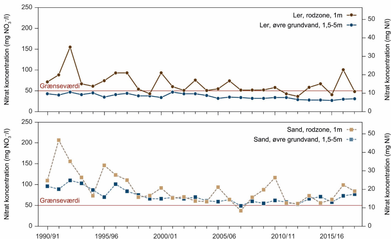
Figur 5.4. Udviklingen i målte nitratkoncentrationer i perioden 1990/91 til 2017/18 i rodzonevand og det øvre grundvand i tre lerjords- og to sandjordsoplande (LOOP). Grænseværdien angiver EU's krav til maksimal nitratkoncentration i grundvand (Blicher-Mathiesen et al. 2019).
