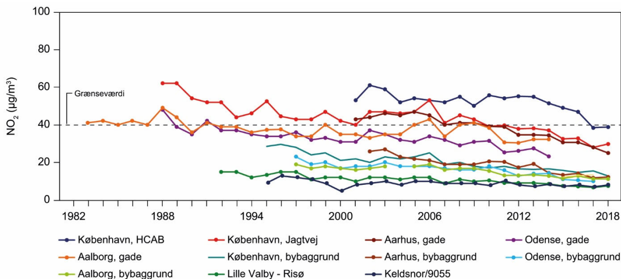
Figur 4.1. Graferne viser tidsserier for årlige gennemsnitsværdier af NO 2 for de forskellige målestationer. Grænseværdien er 40 µg/m 3 og trådte i kraft i 2010 (Ellermann et al. 2019).
