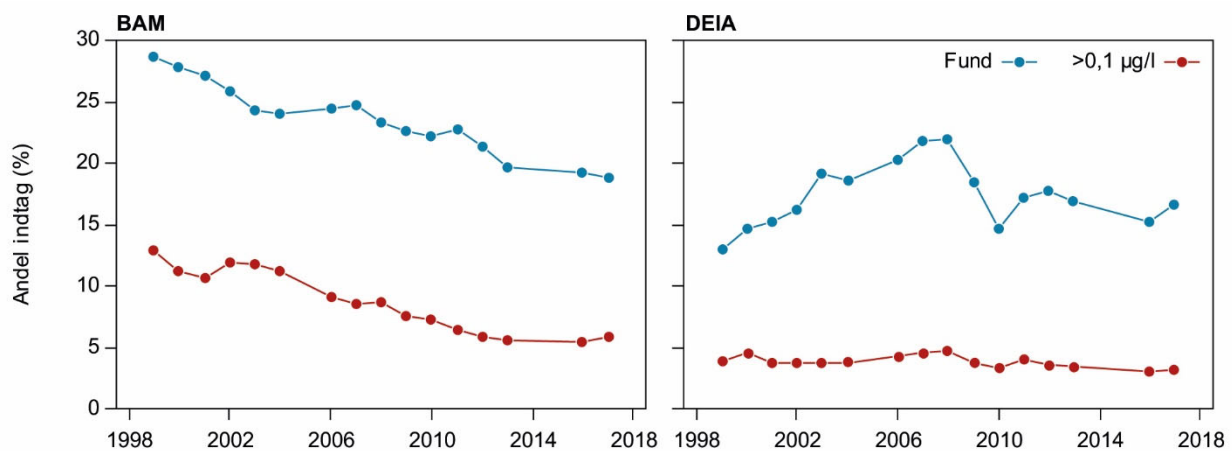
Figur 5.6 Tidslig udvikling i fund af BAM og DEIA i "den faste kerne" af indtag i grundvandsovervågningen. Hvert år repræsenterer opgørelser af andelen af indtag, hvor pesticidet er påvist mindst én gang inden for en treårs periode (forudgående, aktuelle og efterfølgende år) (Thorling et al, 2019).
