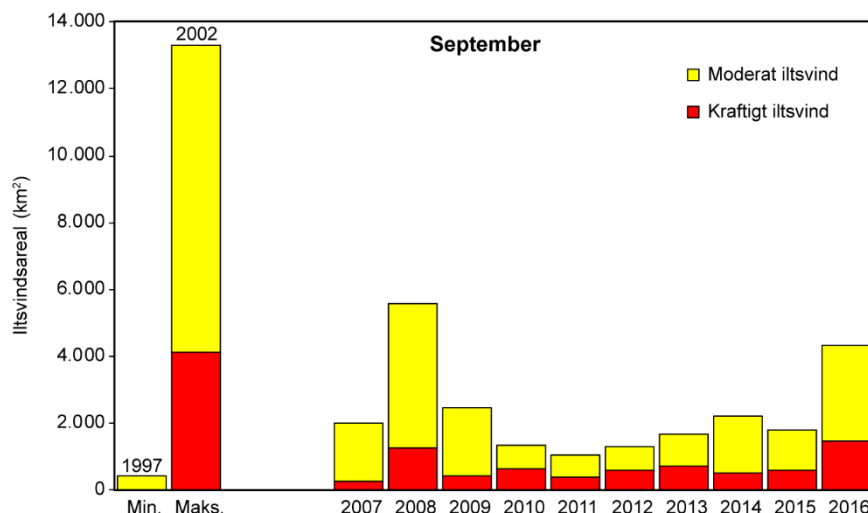
Figur 8.2. Udviklingen i arealet af moderat iltsvind (2-4 mg/l) og kraftigt iltsvind (< 2 mg/l) i september i de indre danske farvande for perioden 2007-2016 samt den største og mindste registrerede arealudbredelse i overvågningsperioden 1989-2016 (Hansen (red) 2018).
