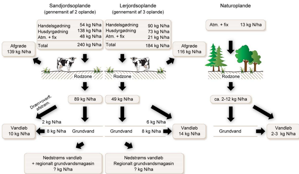
Figur 1.4. Skematiskering af kvælstofkredsløbet i henholdsvis dyrkede lerjords- og sandjordsoplande samt for naturoplande (Blicher-Mathiesen et al. 2018).
