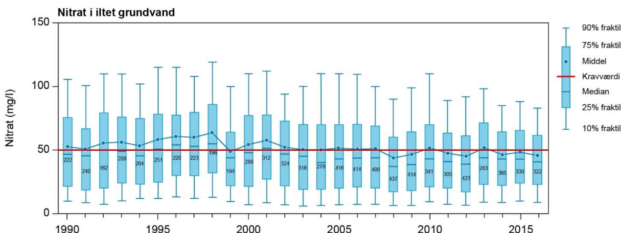
Figur 5.3. Udviklingen i det iltholdige grundvands nitratinhold i grundvandsovervågningen vist for hvert prøvetagningsår i perioden 1990-2016. Beregnet på baggrund af det gennemsnitlige nitratinhold per indtag per år. Antal af indtag er angivet for hvert år (Thorling et al. 2018).
