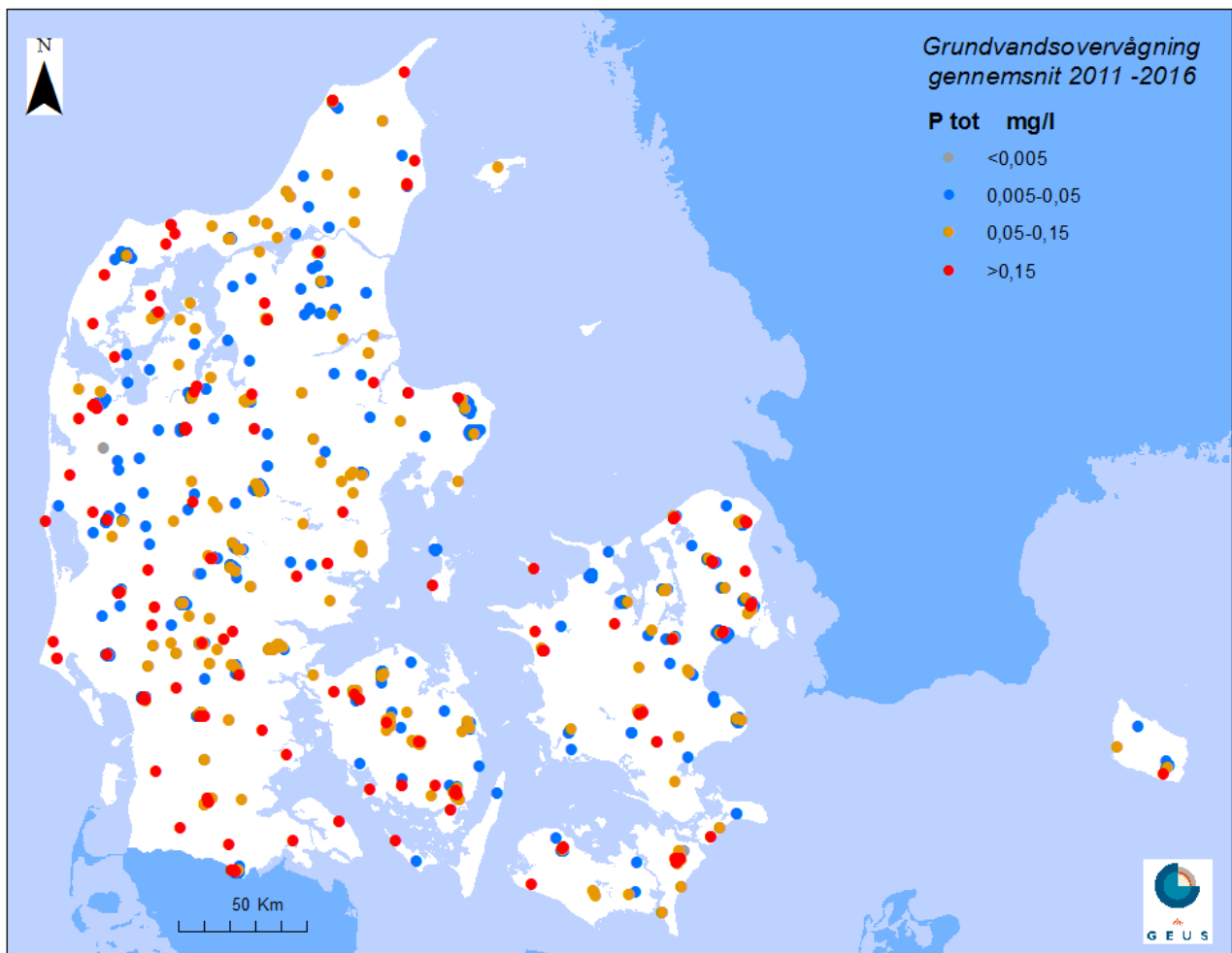
Figur 2.5. Geografisk fordeling af det gennemsnitlige totalfosfor (Ptot) i grundvand i 1127 GRUMO-indtag for perioden 2011-2016. De højeste værdier er udtegnat øverst.
