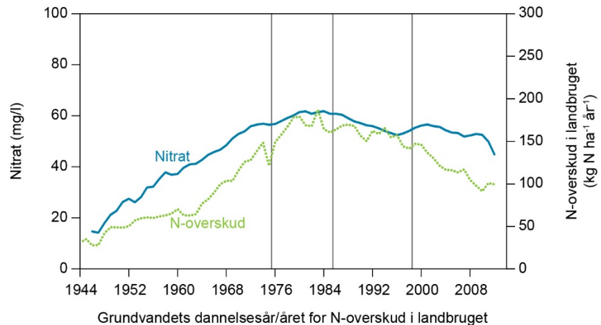
Figur 5.5. Gennemsnitligt nitratindehold som 5-års glidende gennemsnit af i iltet grundvand i forhold til året for grundvandets dannelse og overskud af kvælstof fra landbrugsproduktionen, dvs. den faktuelle nationale kvælstofbalance beregnet for hvert år (Thorling et al. 2018).
